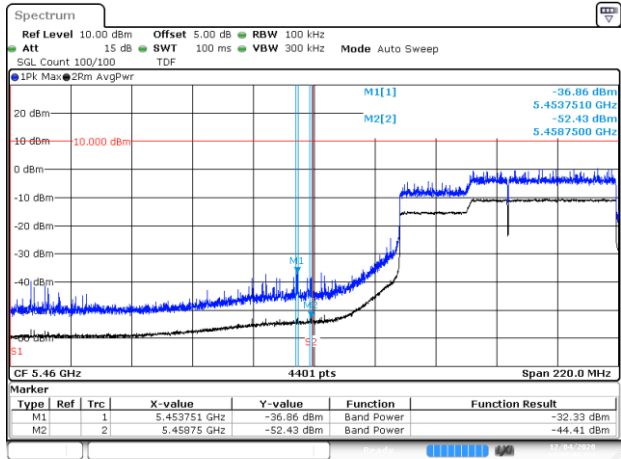
BE-R-LOW, MIMO-A, 802.11ax160-HE0, Ch114
