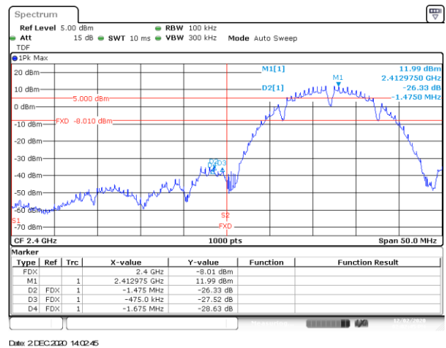
BE-NR, SISO-A, 802.11b-1Mbps, Ch1
