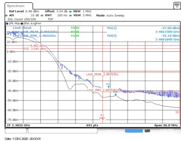
BE-R-HIGH, SISO-A, 802.11b-1Mbps, Ch12
