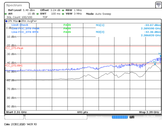
BE-R-LOW, SISO-A, 802.11b-1Mbps, Ch1
