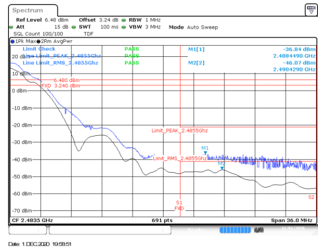
BE-R-HIGH, SISO-A, 802.11b-1Mbps, Ch11
