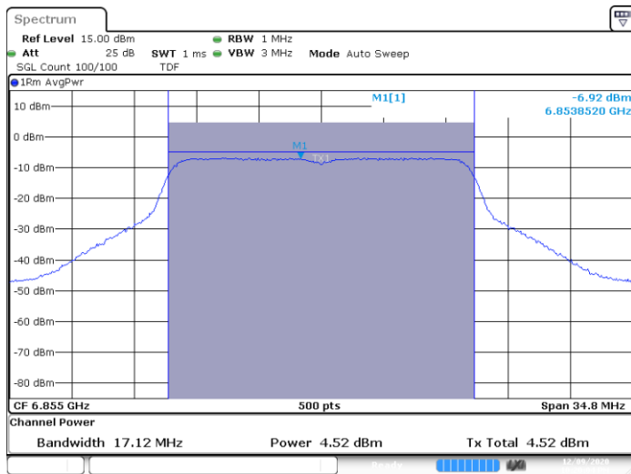
SISO A-802.11a-20MHz-Ch181-6855MHz-6
