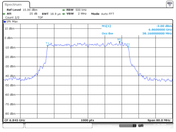
UNII7 MIMO B 802.11ax40 ch179 6845MHz 99%
