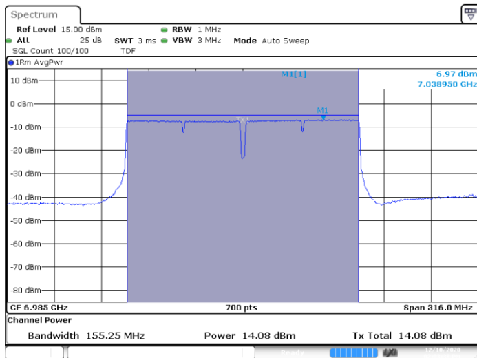
SISO A-802.11ac-160MHz-Ch207-6985MHz-VHT0
