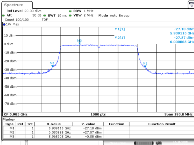
UNI15 MIMO A 802.11ac80 ch7 5985MHz 26dB
