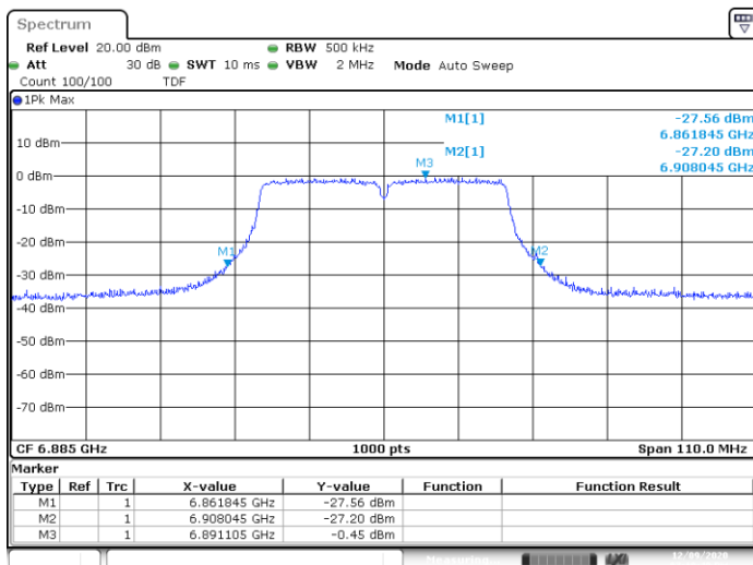
UNII8 SISO A 802.11n40 ch187 6885MHz 26dB
