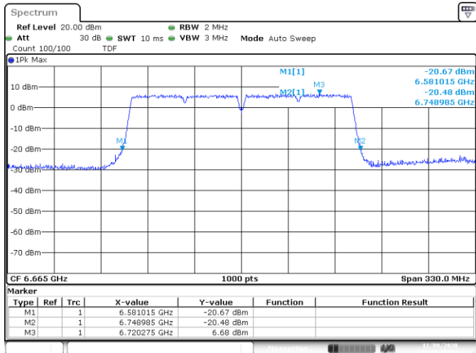
UNI17 SISO A 802.11ac160 ch143 6665MHz 26dB
