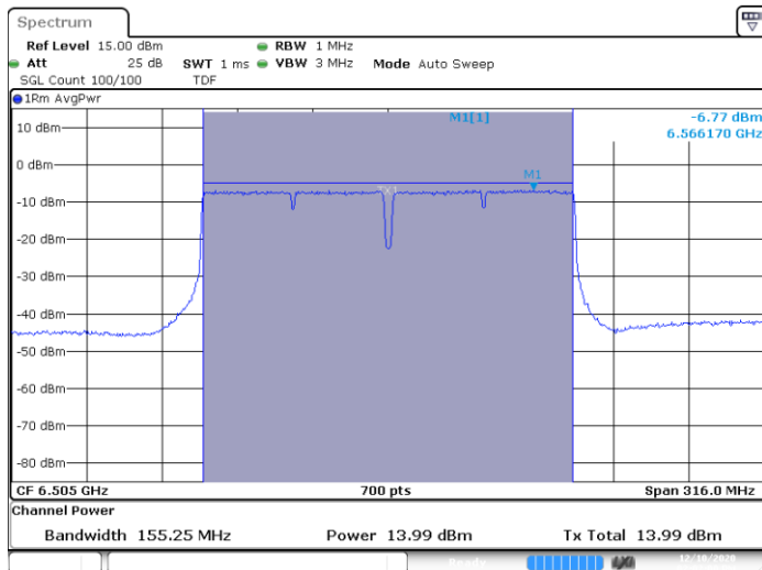
SISO A-802.11ac-160MHz-Ch111-6505MHz-VHT0
