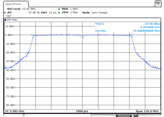
UNI15 MIMO A 802.11ac80 ch7 5985MHz 99%
