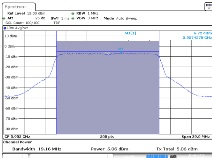
SISO A-802.11ax-20MHz-Ch1-5955MHz-HE0
