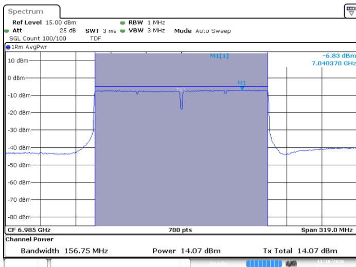
SISO A-802.11ax-160MHz-Ch207-6985MHz-HE0
