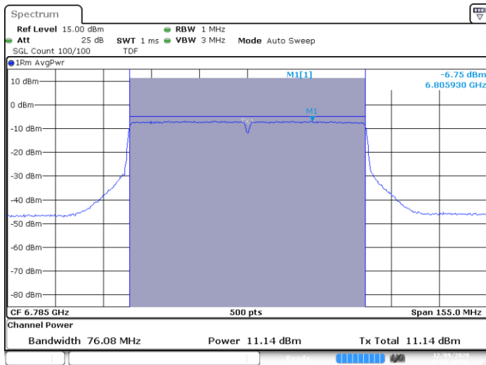
SISO A-802.11ac-80MHz-Ch167-6785MHz-VHT0
