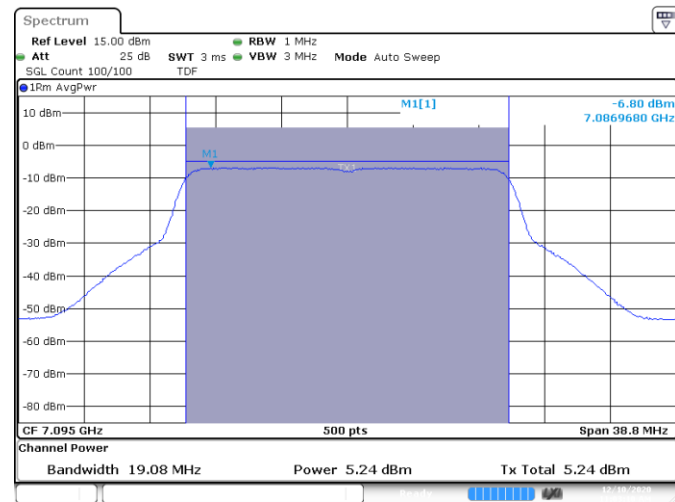
SISO B-802.11ax-20MHz-Ch229-7095MHz-HE0
