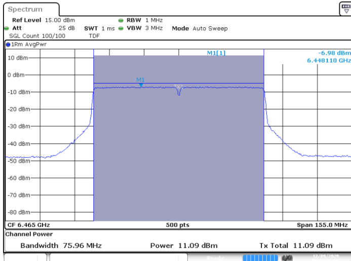
SISO A-802.11ac-80MHz-Ch103-6465MHz-VHT0
