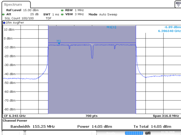
SISO A-802.11ac-160MHz-Ch79-6345MHz-VHT0
