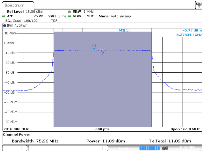
SISO A-802.11ac-80MHz-Ch87-6385MHz-VHT0
