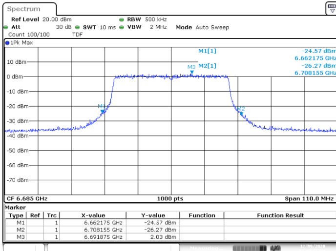
UNII7 SISO A 802.11ax40 ch147 6685MHz 26dB
