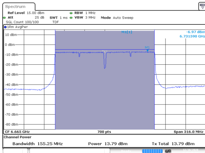
SISO A-802.11ac-160MHz-Ch143-6665MHz-VHT0
