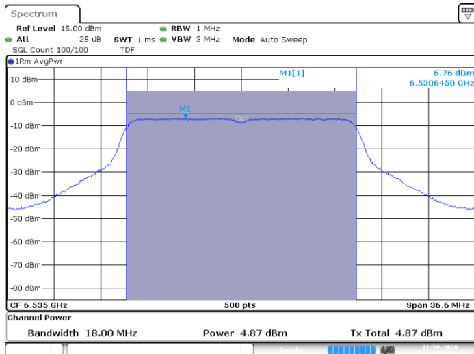
SISO A-802.11n-20MHz-Ch117-6535MHz-HT0
