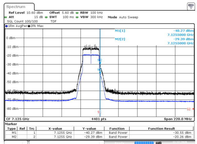
BE-NR-HIGH, MIMO-B, 802.11ax20-HE0, Ch233
