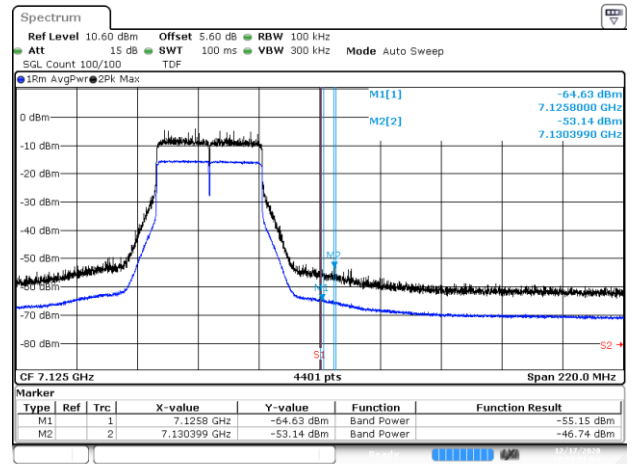
BE-NR-HIGH, MIMO-B, 802.11ax40-HE0, Ch227
