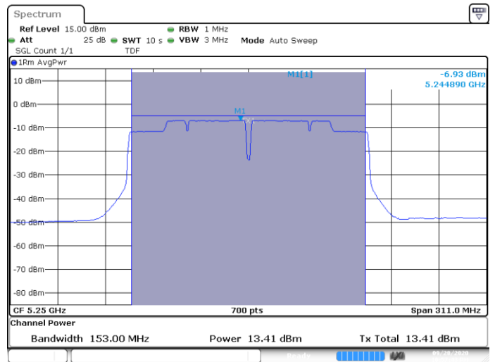
MIMO B-802.11ac-160MHz-Ch50-5250MHz-VHT0
