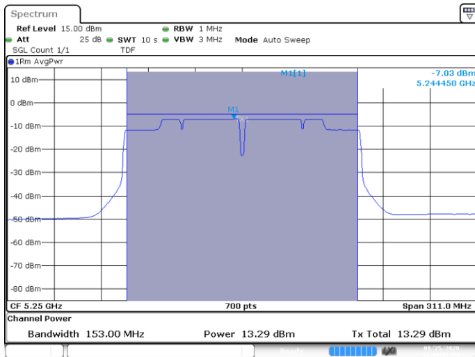
MIMO A-802.11ac-160MHz-Ch50-5250MHz-VHT0
