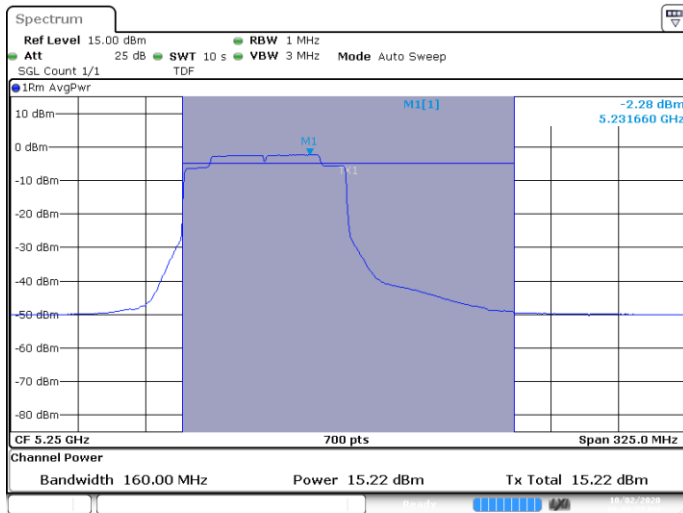
MIMO A-802.11ax-160MHz-Ch50-5250MHz-HE0-996/67
