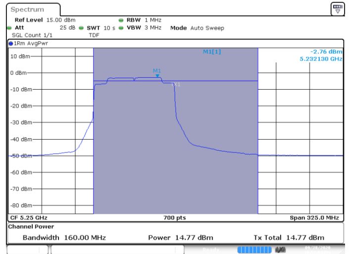
MIMO B-802.11ax-160MHz-Ch50-5250MHz-HE0-996/67
