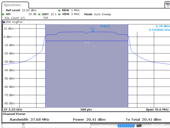
MIMO A-802.11ax-40MHz-Ch46-5230MHz-HE0
