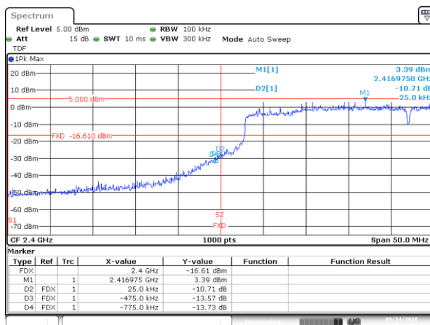
BE-NR, SISO-A, 802.11ax40-HE0, Ch1
