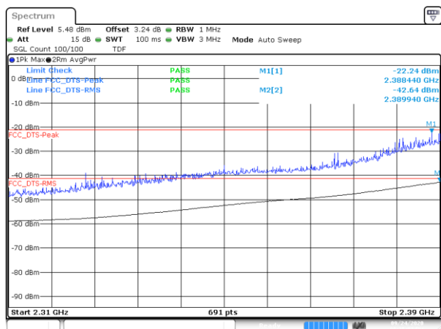
BE-R-LOW, SISO-A, 802.11ax40-HE0, Ch1
