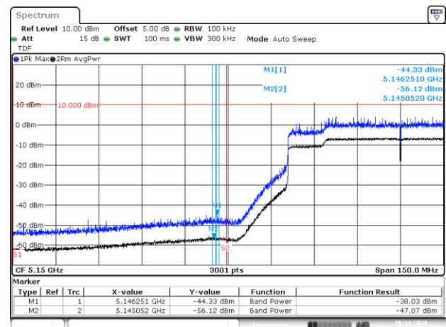
BE-R-LOW, MIMO-A, 802.11ax80-HE0, Ch42
