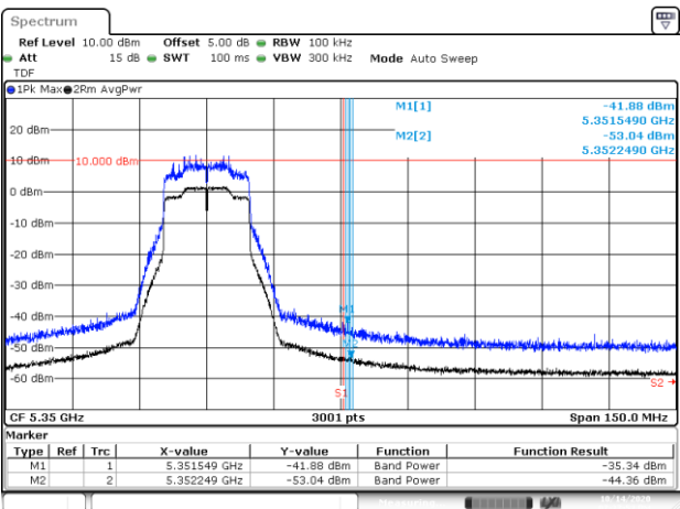
BE-R-HIGH, SISO-A, 802.11ax20-HE0, Ch64
