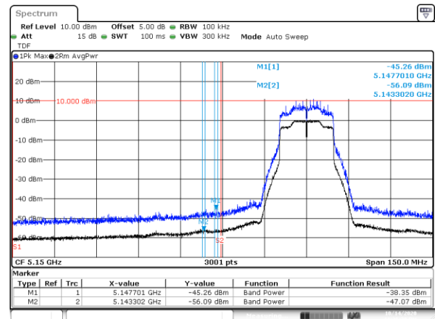
BE-R-LOW, MIMO-A, 802.11ax20-HE0, Ch36
