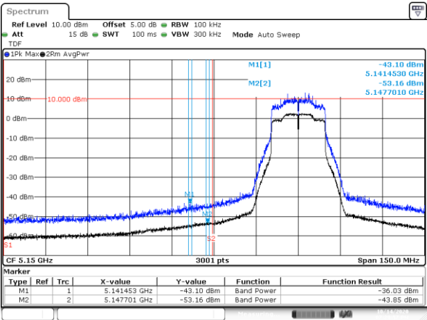
BE-R-LOW, SISO-A, 802.11ax20-HE0, Ch36
