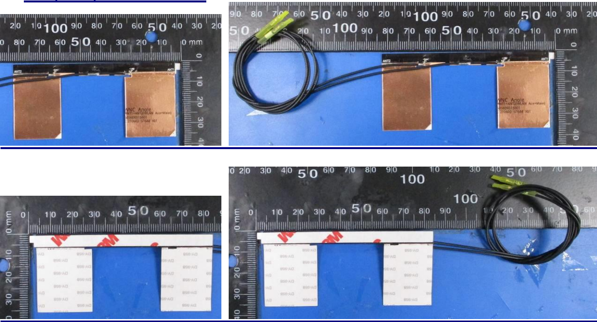
Tx1 (AUX) Antenna Photo:
