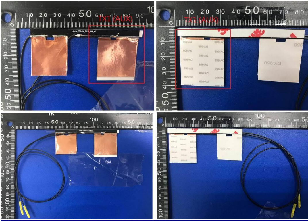
Tx1 (AUX) Antenna Photo:
