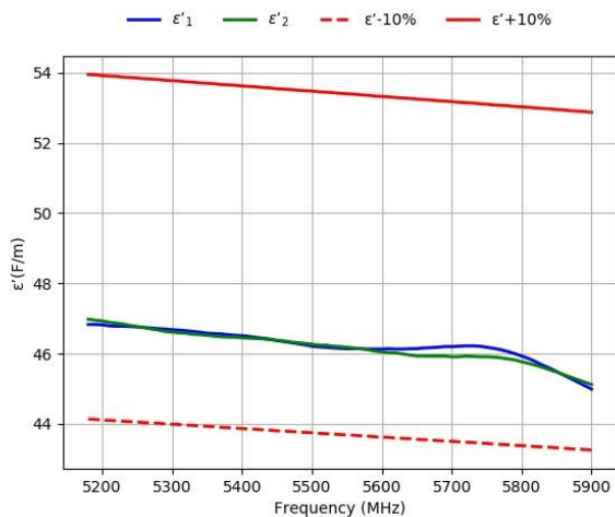
Permittivity
