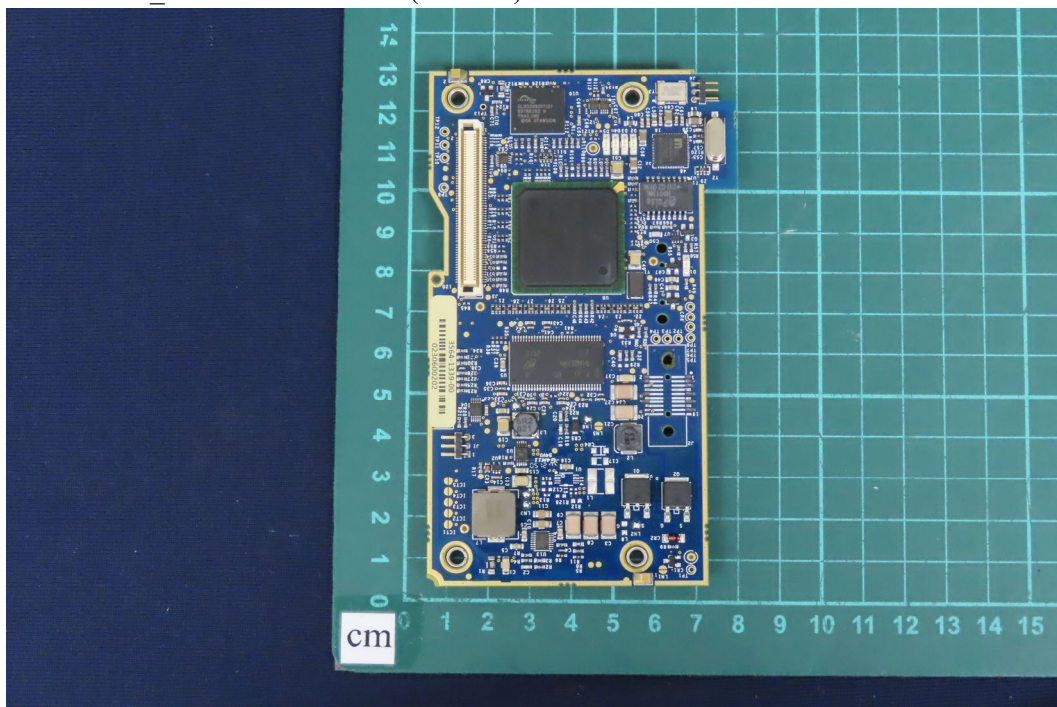
(62) EUT Photo_M/N: 3571-0100-5x (TMVCI)
