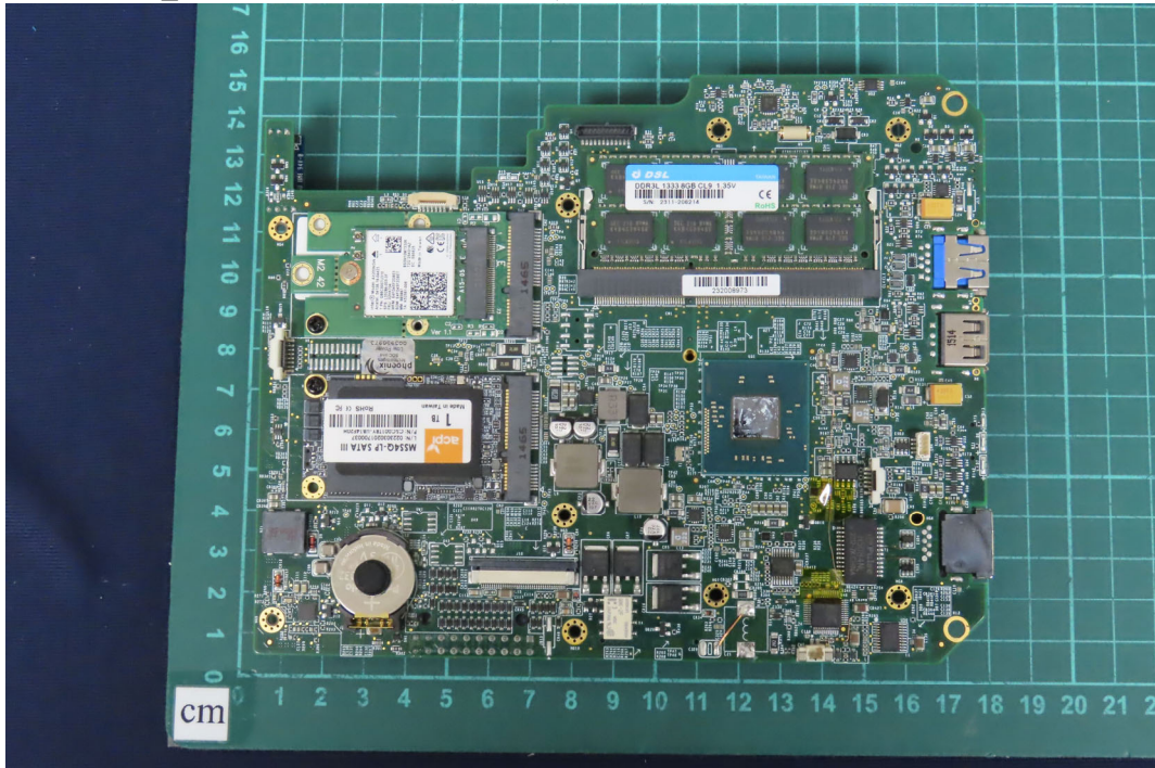
(67) EUT Photo_M/N: 3571-0100-5x (TMVCI)
