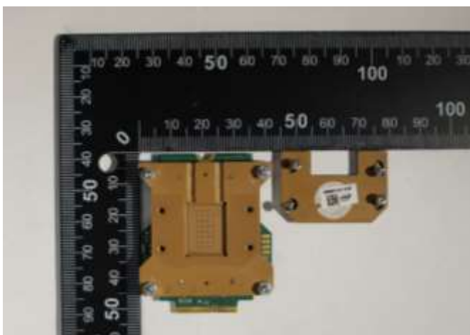
Socket
