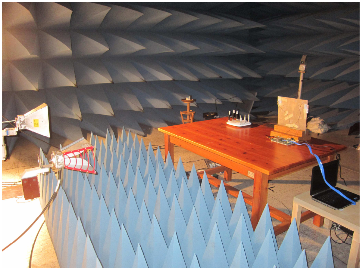
Fig. 3. Test setup
