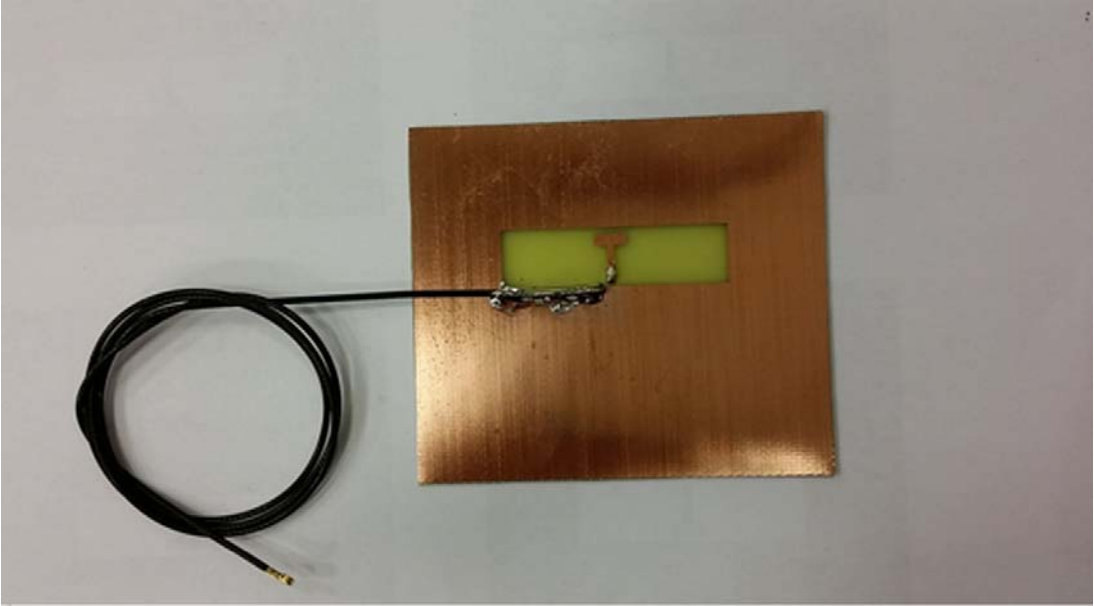
(5) EUT Photo
