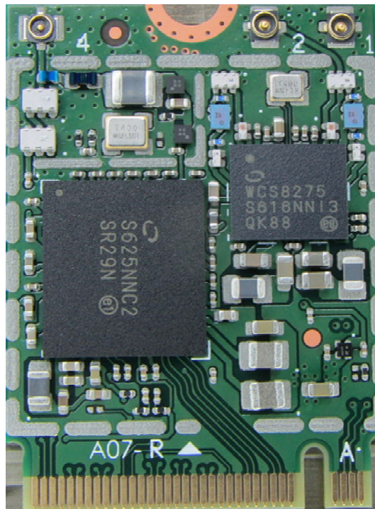
WiFi Module
