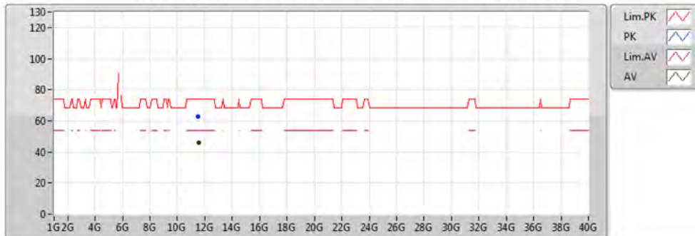
RE TX above 1GHz;Band:5.8G;VHT40,BF;BWch:40MHz;Nss:1,(M0);Nant:4;Ch:5755MHz;TX
