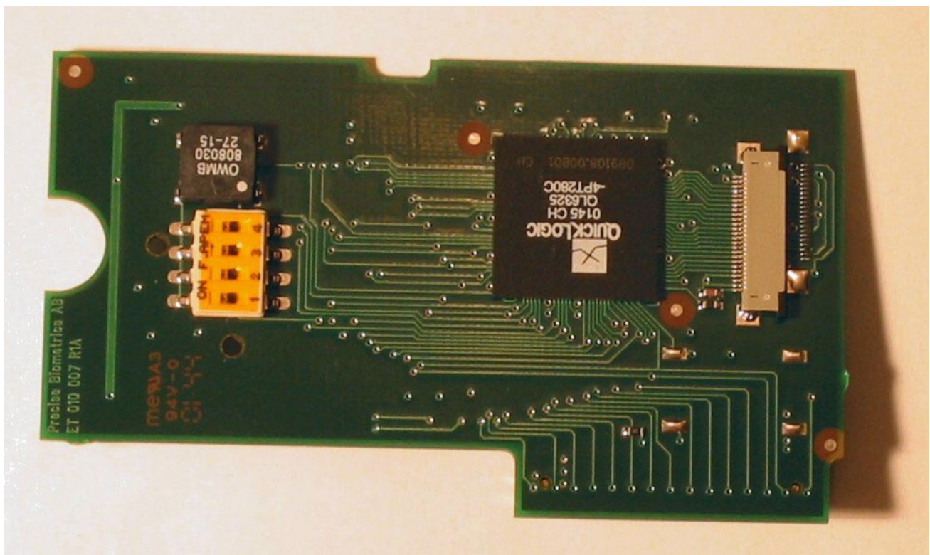
Front CPU PCA
