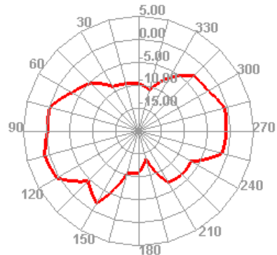
2450.000MHz E1
