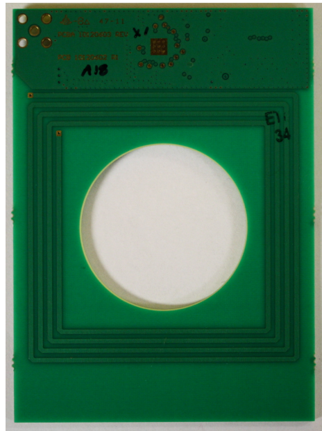
RFID PCBA - Top
