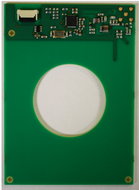
RFID PCBA – Bottom
