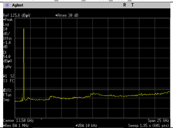
2437MHz_20MHz_n-mode_avg_Ant B
