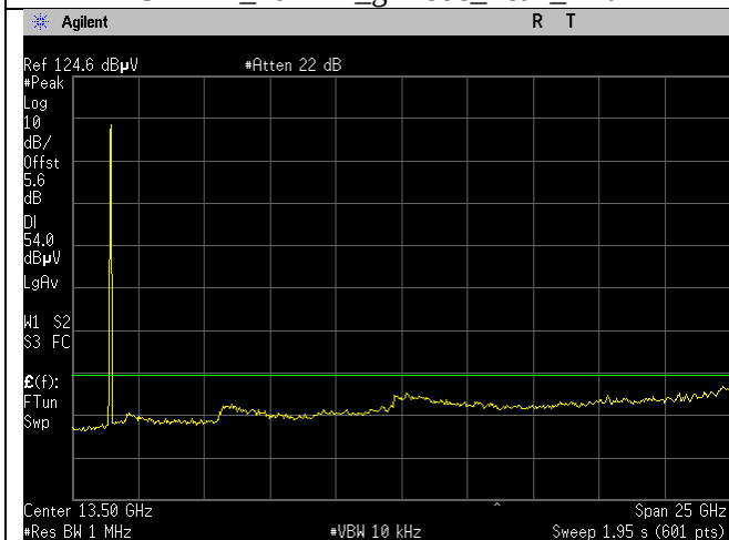
2437MHz_20MHz_g-mode_avg_Ant A
