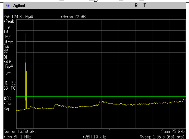
2437MHz_20MHz_g-mode_avg_Ant B
