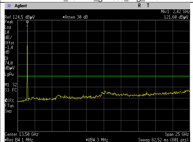
2412MHz_20MHz_n-mode_Peak_Ant B
