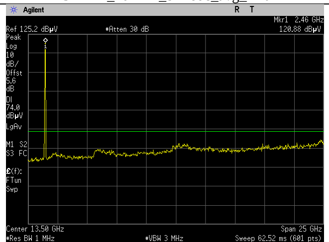
2437MHz_20MHz_g-mode_Peak_Ant B
