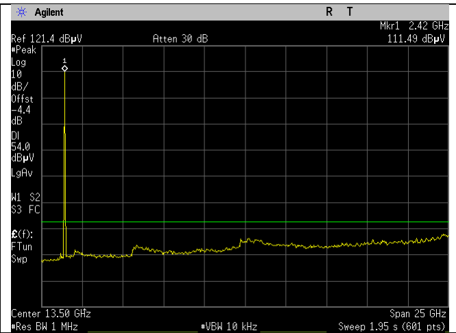
2412MHz_20MHz_g-mode_avg_Ant B
