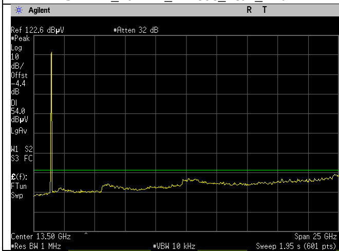
2437MHz_20MHz_n-mode_avg_Ant A
