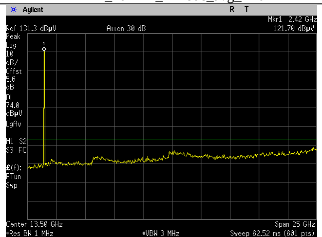
2437MHz_20MHz_b-mode_Peak_Ant B
