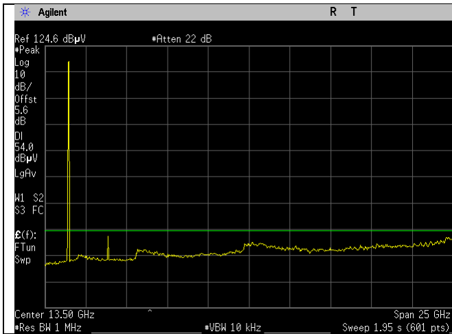
2437MHz_20MHz_b-mode_avg_Ant A
