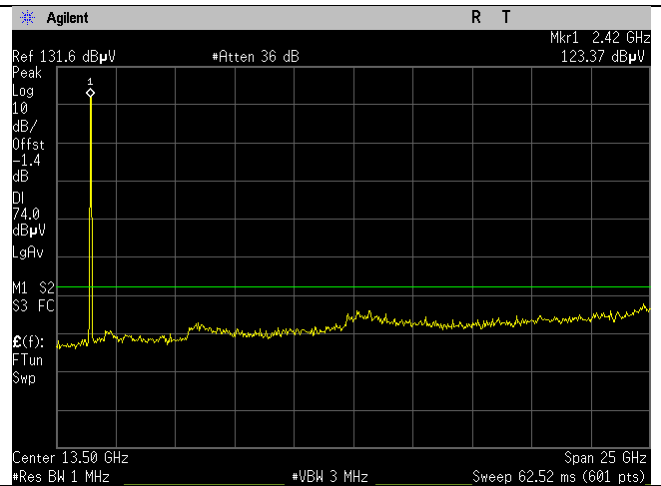
2437MHz_20MHz_n-mode_Peak_Ant B
