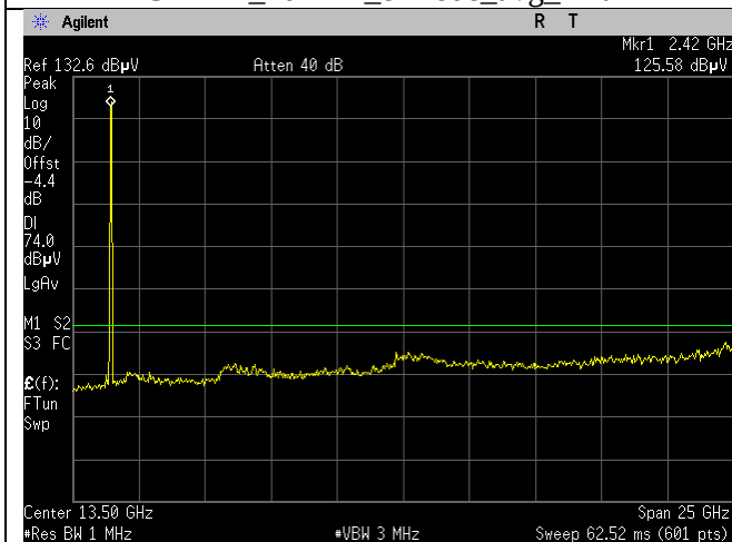
2437MHz_20MHz_g-mode_Peak_Ant A
