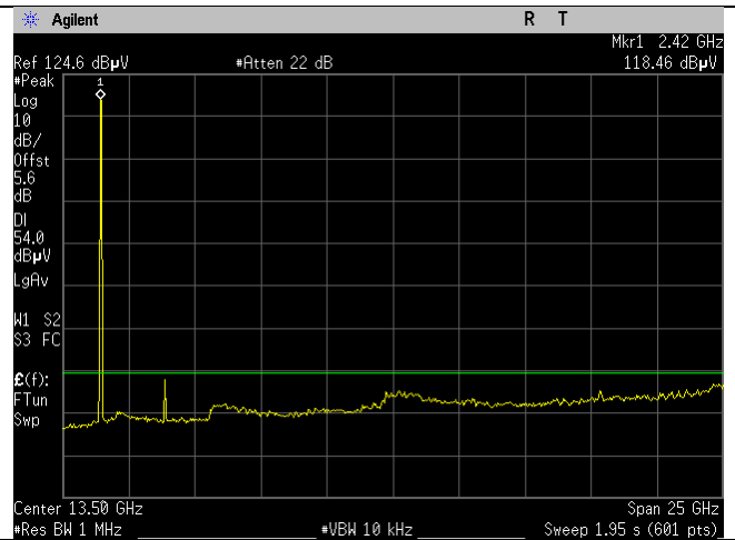
2437MHz_20MHz_b-mode_avg_Ant B
