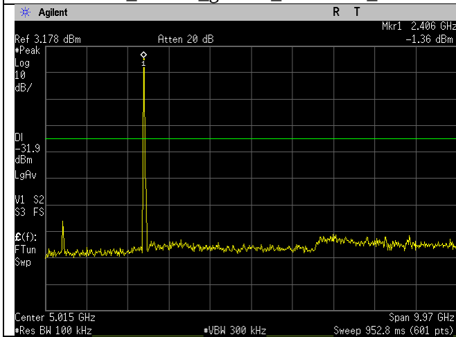
2412MHz_20MHz_g-mode_30MHz-10GHz_Ant A
