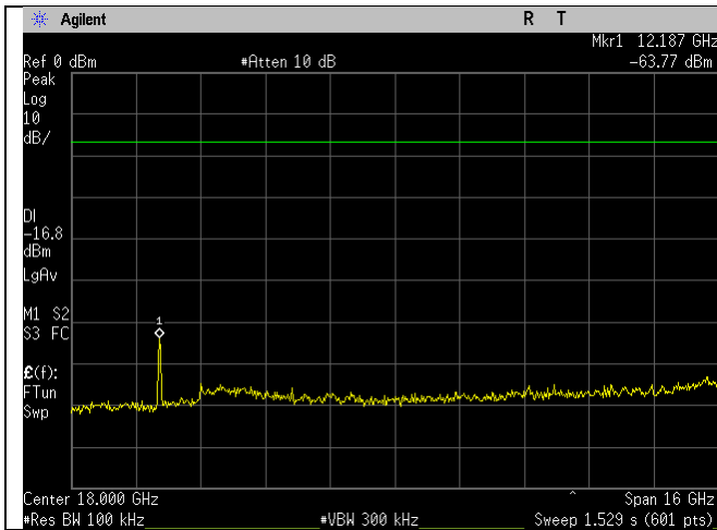
2437MHz_20MHz_g-mode_10-26GHz_Ant A
