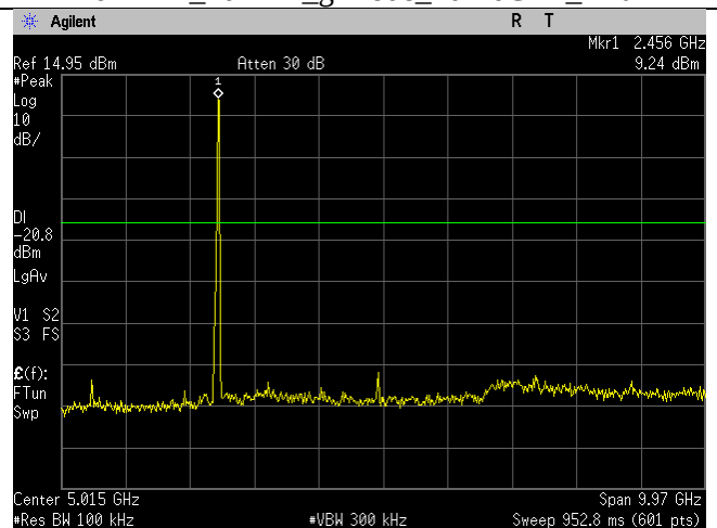
2462MHz_20MHz_g-mode_30MHz-10GHz_Ant B
