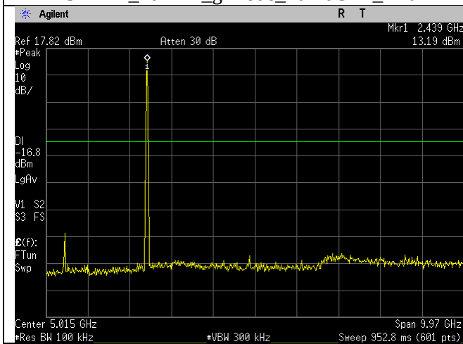
2437MHz_20MHz_g-mode_30MHz-10GHz_Ant A
