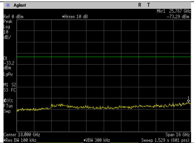
2437MHz_20MHz_g-mode_10-26GHz_Ant B
