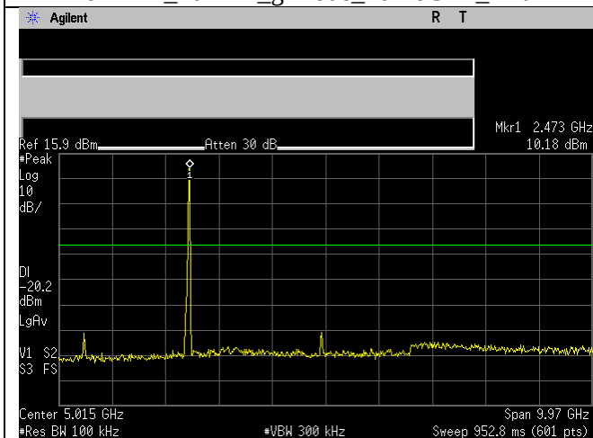
2462MHz_20MHz_g-mode_30MHz-10GHz_Ant A
