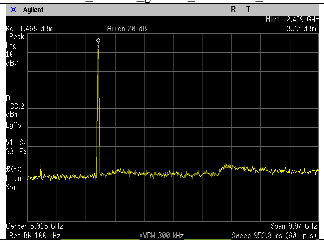
2437MHz_20MHz_g-mode_30MHz-10GHz_Ant B
