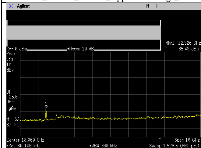
2462MHz_20MHz_g-mode_10-26GHz_Ant A
