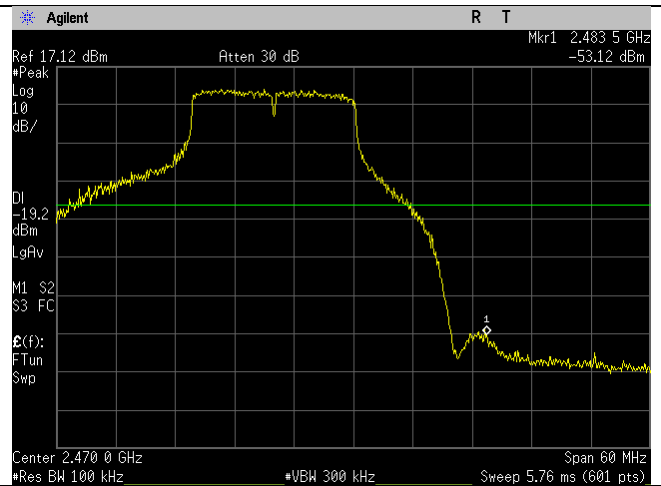
2462MHz_20MHz_g-mode_Upper Band Edge_Ant B
