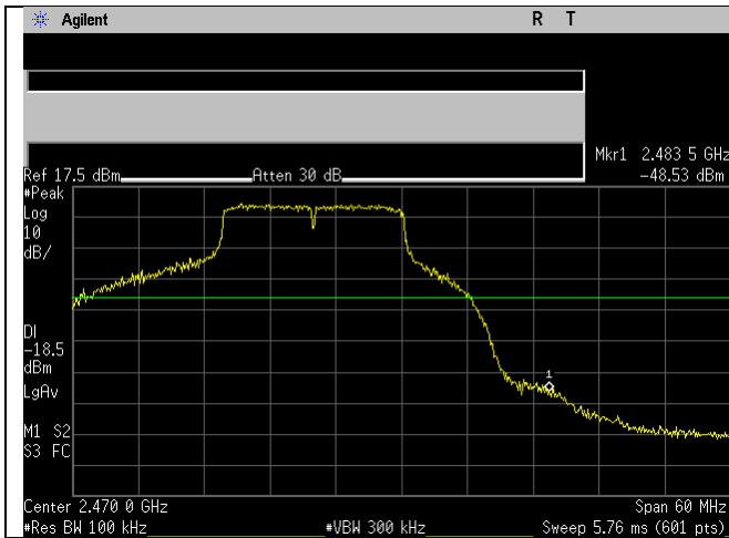
2462MHz_20MHz_g-mode_Upper Band Edge_Ant A
