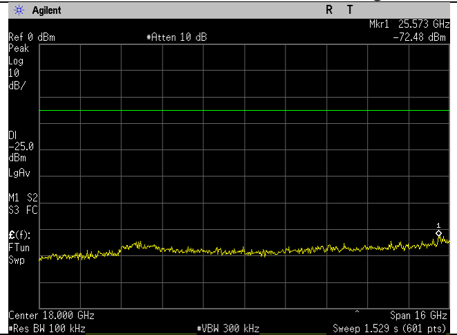
2412MHz_20MHz_g-mode_10-26GHz_Ant B
