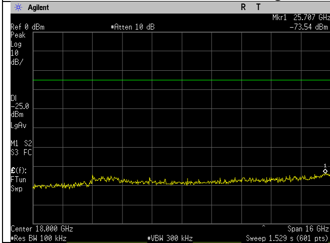
2412MHz_20MHz_g-mode_10-26GHz_Ant A
