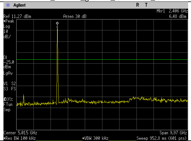
2412MHz_20MHz_g-mode_30MHz-10GHz_Ant B
