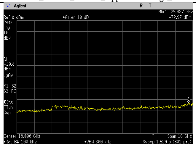
2462MHz_20MHz_g-mode_10-26GHz_Ant B
