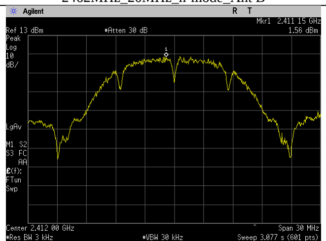
2412MHz_20MHz_b-mode_Ant B
