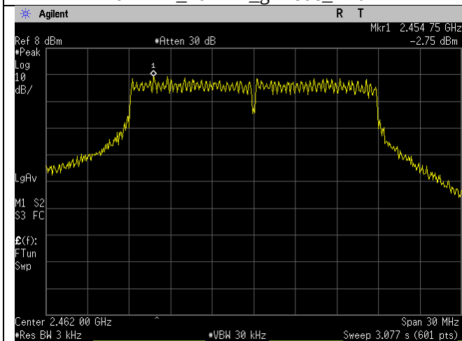
2462MHz_20MHz_n-mode_Ant A
