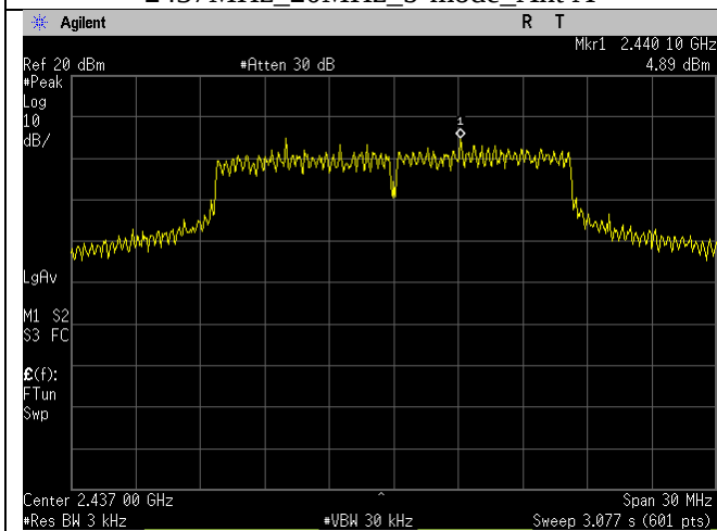
2437MHz_20MHz_g-mode_Ant A
