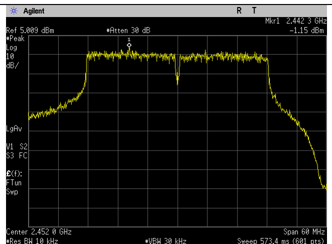
2452MHz_40MHz_n-mode_Ant B
