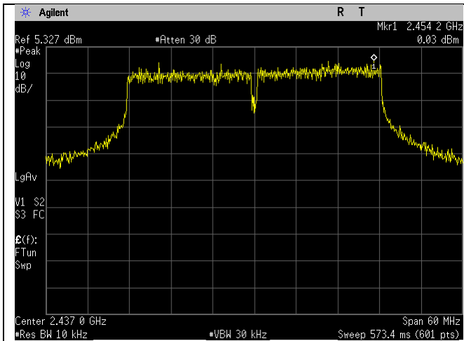
2437MHz_40MHz_n-mode_Ant A
