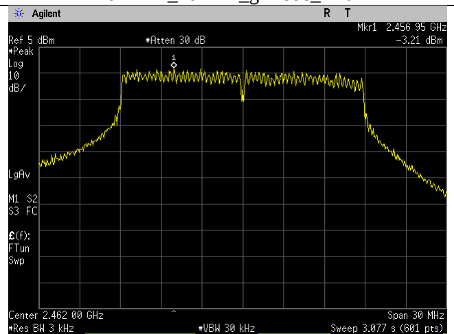
2462MHz_20MHz_n-mode_Ant B
