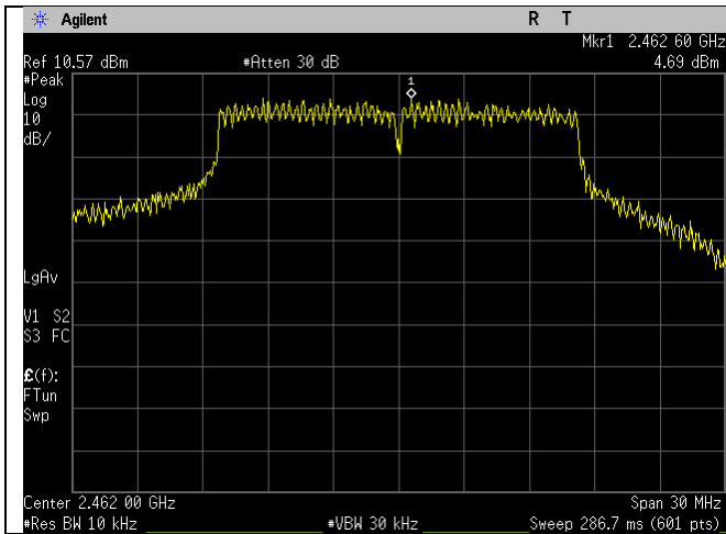
2462MHz_20MHz_g-mode_Ant A
