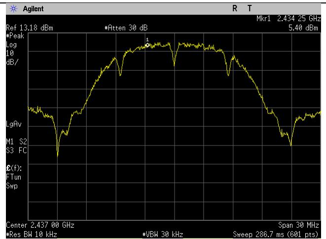
2437MHz_20MHz_b-mode_Ant B
