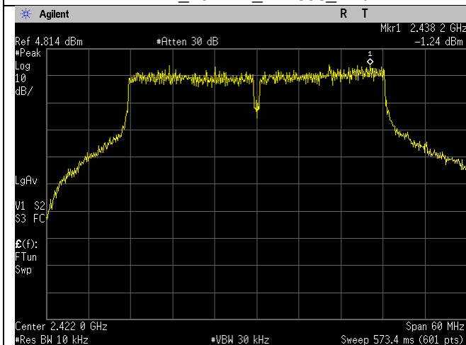
2422MHz_40MHz_n-mode_Ant A
