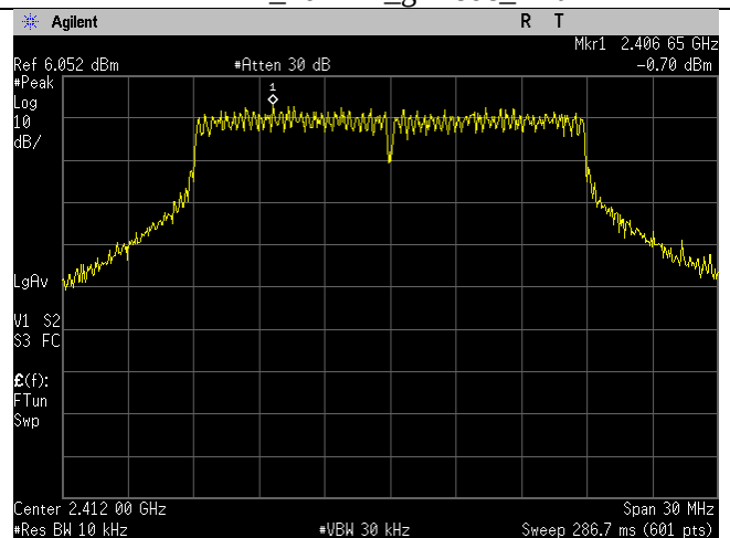
2412MHz_20MHz_n-mode_Ant B
