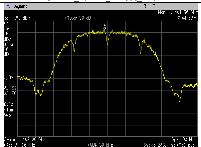
2462MHz_20MHz_b-mode_Ant B
