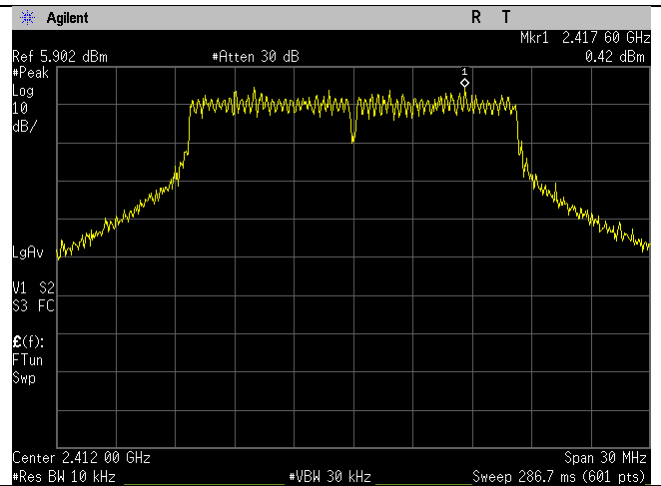
2412MHz_20MHz_g-mode_Ant B
