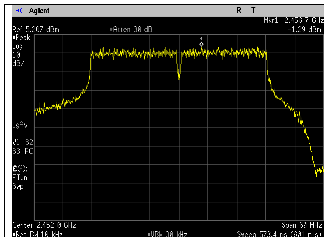
2452MHz_40MHz_n-mode_Ant A
