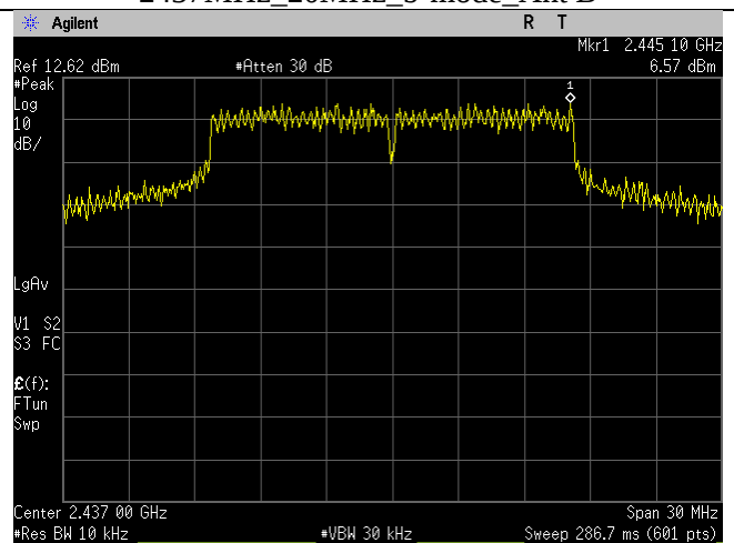
2437MHz_20MHz_g-mode_Ant B
