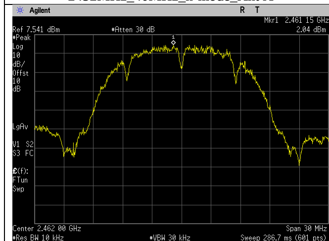
2462MHz_20MHz_b-mode_Ant A
