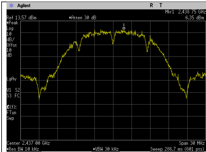
2437MHz_20MHz_b-mode_Ant A
