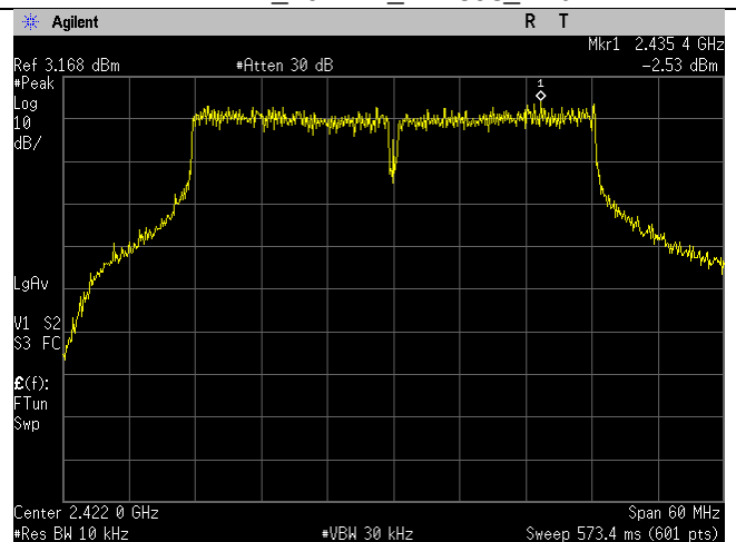
2422MHz_40MHz_n-mode_Ant B
