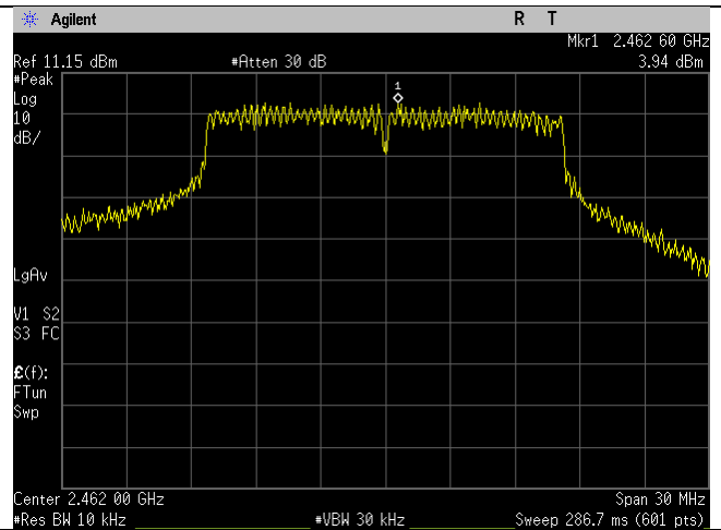
2462MHz_20MHz_g-mode_Ant B
