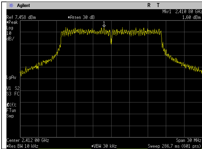
2412MHz_20MHz_g-mode_Ant A
