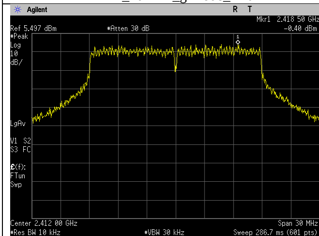
2412MHz_20MHz_n-mode_Ant A
