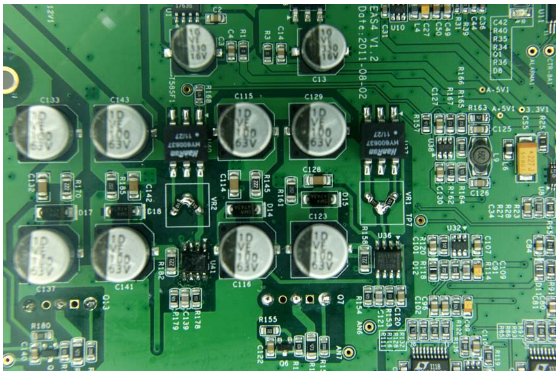
(5) EUT Photo
