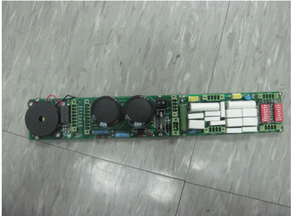
(6) EUT Photo
