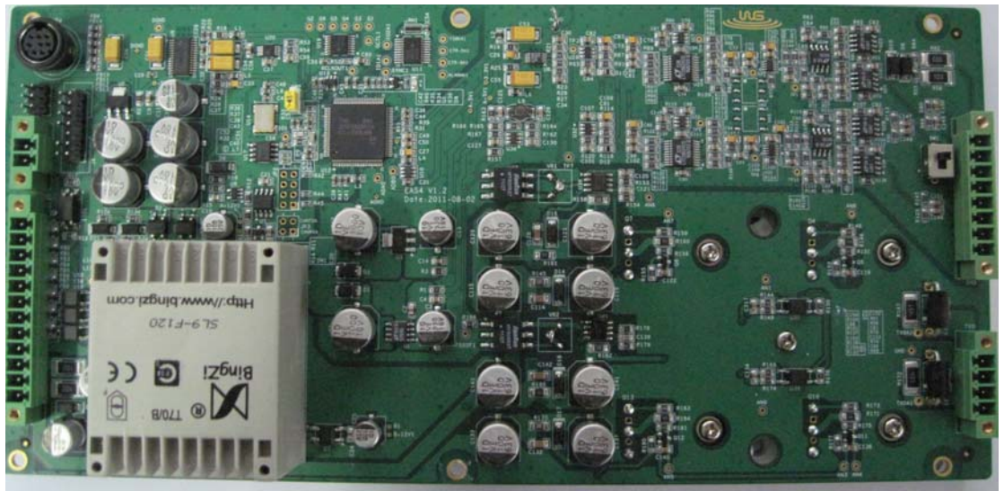
(4) EUT Photo
