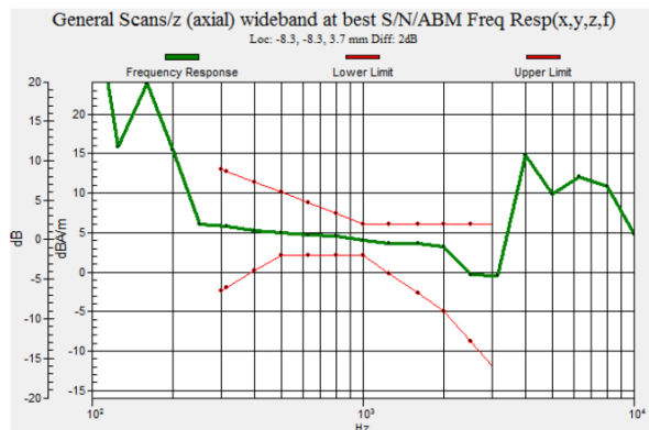
Fig 7.1 GSM850 Ch189
