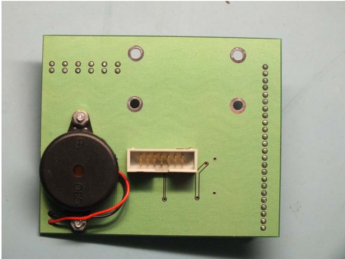
150BP104 Top
