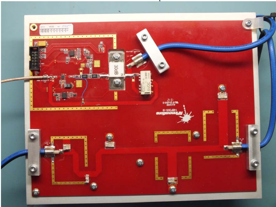
148P305-B Top
