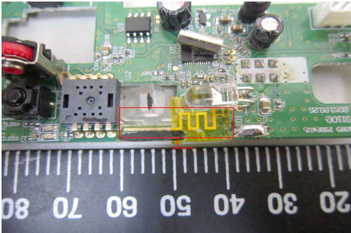
2.4GHz Antenna
