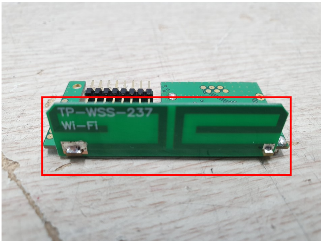
Antenna_WiFi 2.4 GHz
