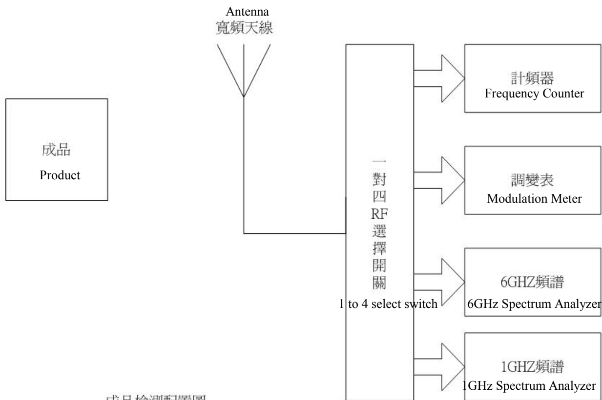
成品檢測配置圖 Product inspection diagram
