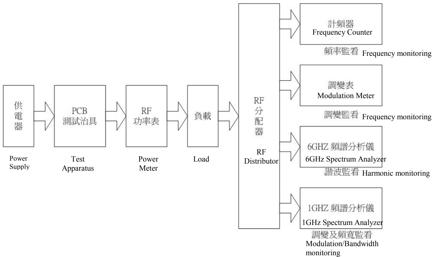
PCB檢測配置圖 PCB Inspection Diagram
