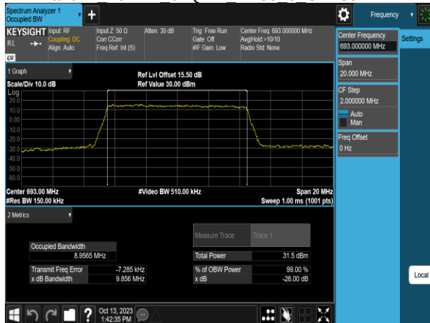
Band71 10MHz 64QAM RB50 0 CH133422
