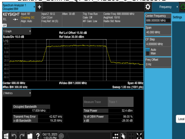
Band71 20MHz QPSK RB100 0 CH133372
