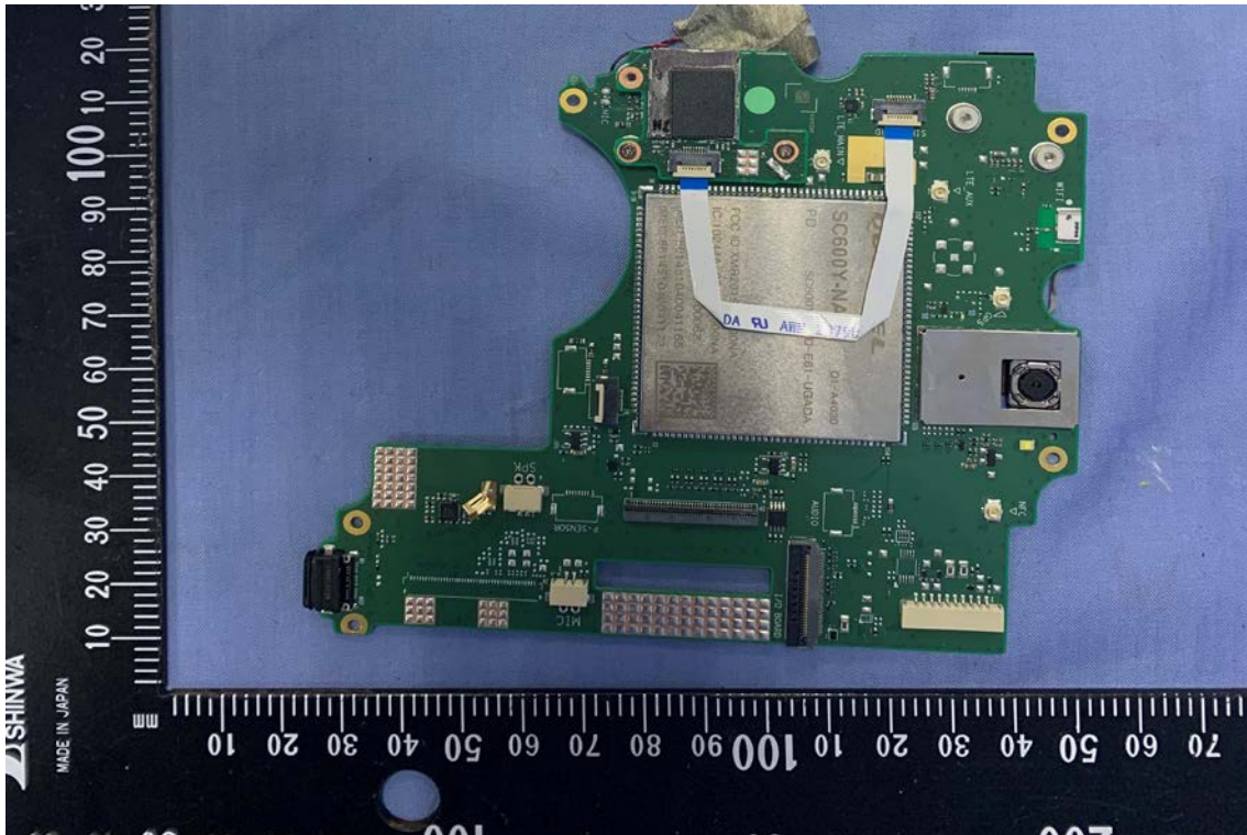
RF IC &amp; Crystal
