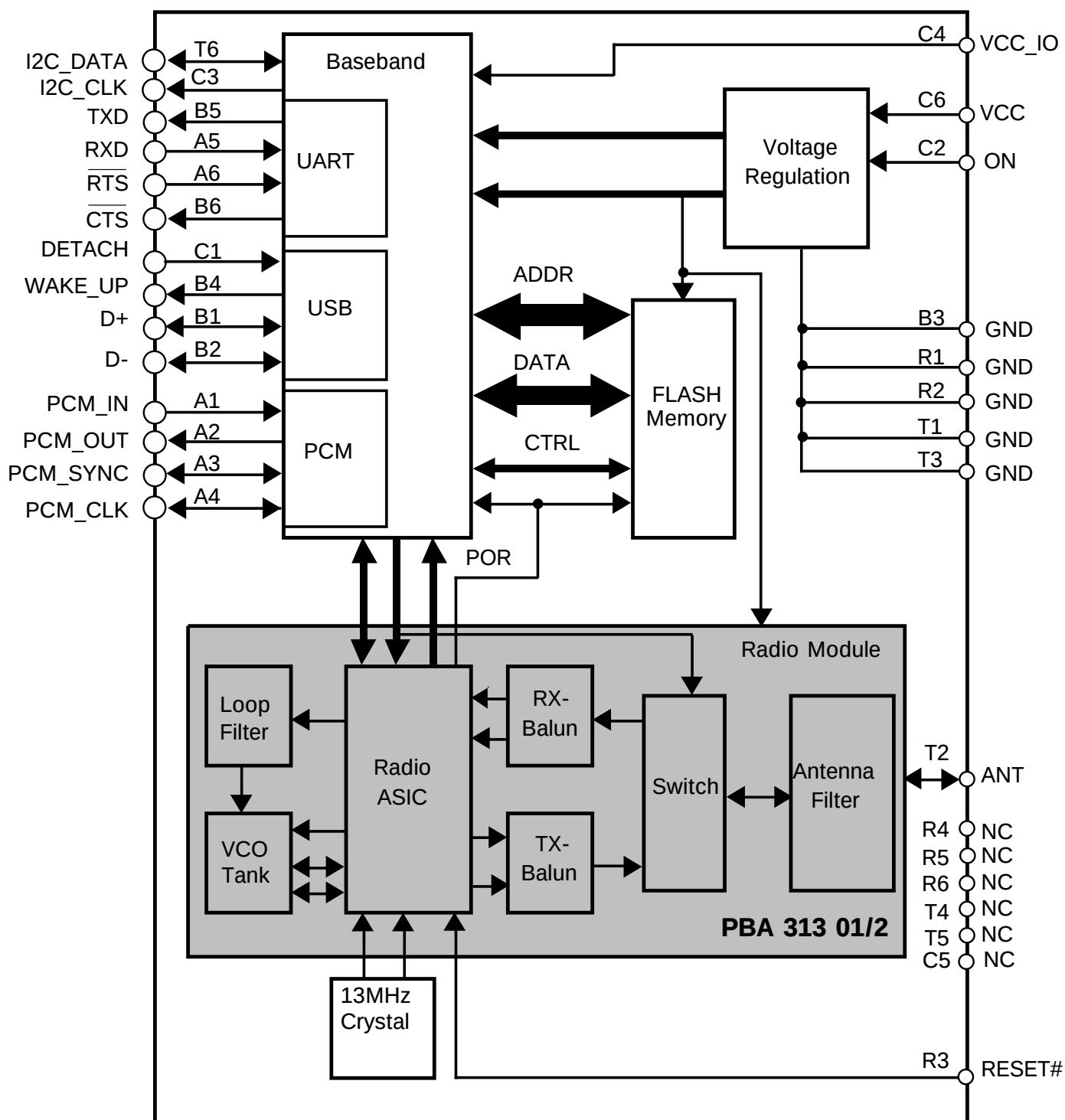
Block diagram for Ericsson Bluetooth modules ROK 101 007 and ROK 101 008
