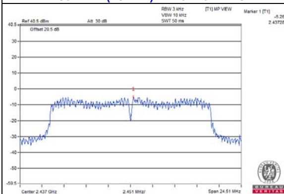
802.11n (20MHz) / Chain 0 : CH6
