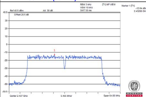
802.11n (40MHz) / Chain 1 : CH6
