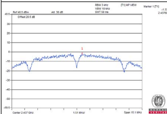
802.11n (20MHz) / Chain 0 : CH6
