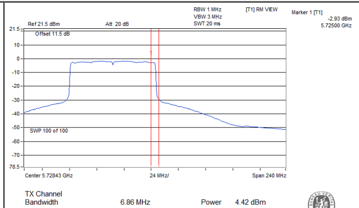
802.11be (EHT80) CDD / Chain 3 : CH 138 (U-NII-3)
