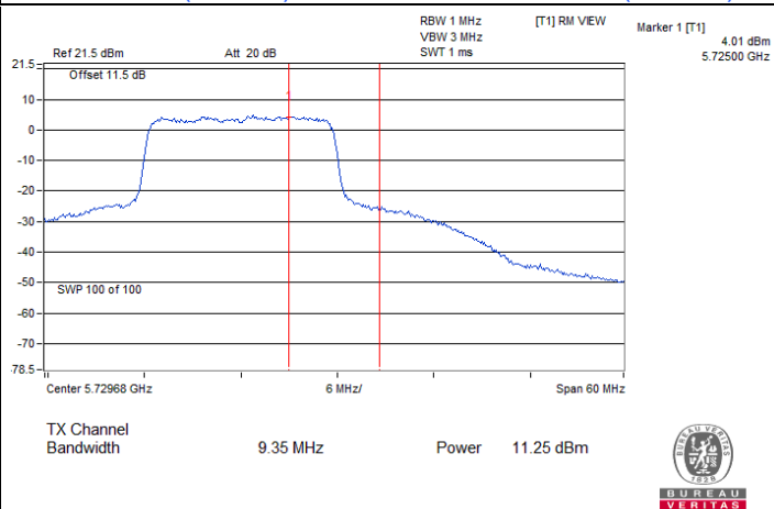
802.11be (EHT20) CDD / Chain 1 : CH 144 (U-NII-3)
