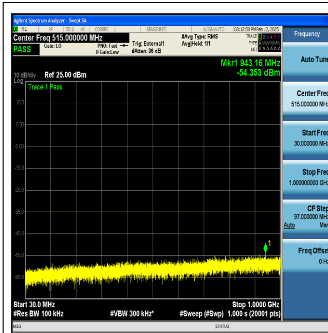
NTNV-n41-PC2-30-100-L-CP-QPSK-Edge_1RB_Left-30-1000-PASS
