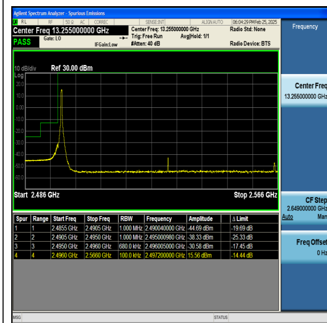
NTNV-n41-PC2-30-70-L-CP-QPSK-Edge_1RB_Left-PASS
