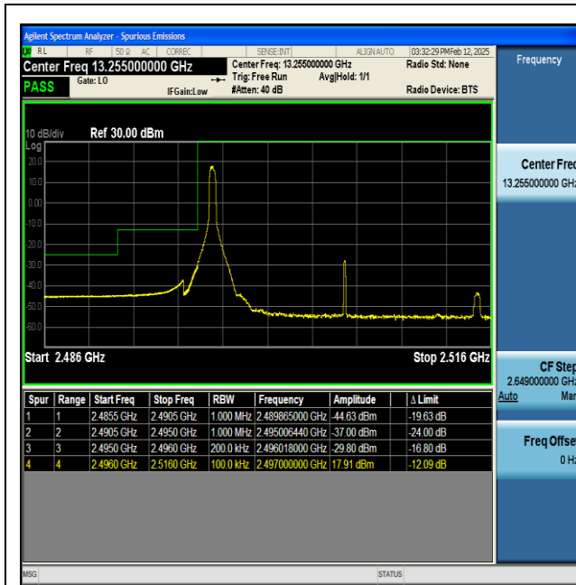
NTNV-n41-PC2-30-20-L-DFT-BPSK-Edge_1RB_Left-PASS
