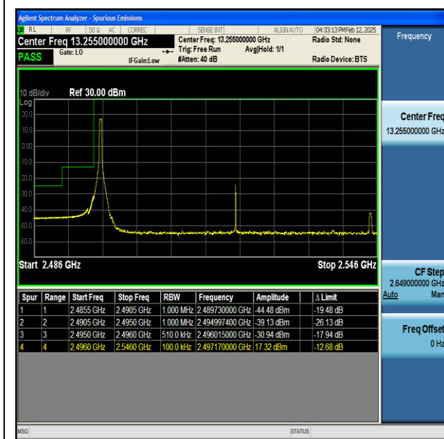
NTNV-n41-PC2-30-50-L-CP-QPSK-Edge_1RB_Left-PASS
