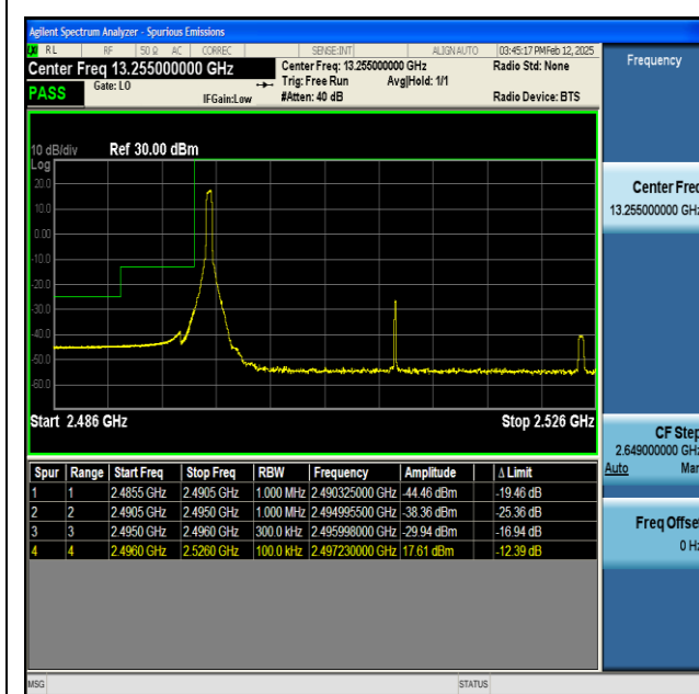
NTNV-n41-PC2-30-30-L-CP-QPSK-Edge_1RB_Left-PASS
