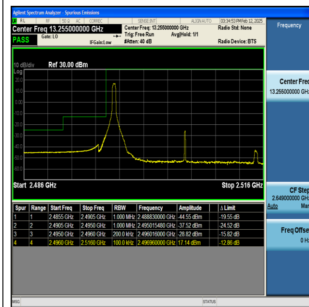
NTNV-n41-PC2-30-20-L-CP-QPSK-Edge_1RB_Left-PASS
