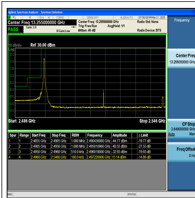
NTNV-n41-PC2-30-50-L-DFT-BPSK-Edge_1RB_Left-PASS
