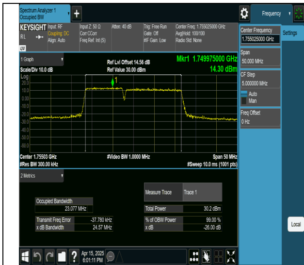
66-66-10MHz-15MHz-QPSK-QPSK-132351-132471-50RB#0-75RB#0-PASS
