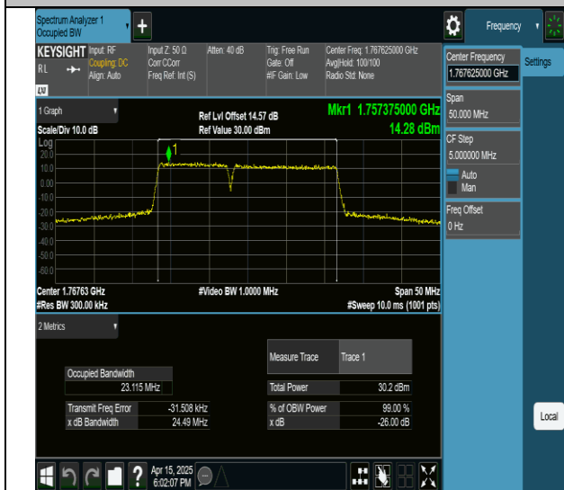
66-66-10MHz-15MHz-QPSK-QPSK-132477-132597-50RB#0-75RB#0-PASS
