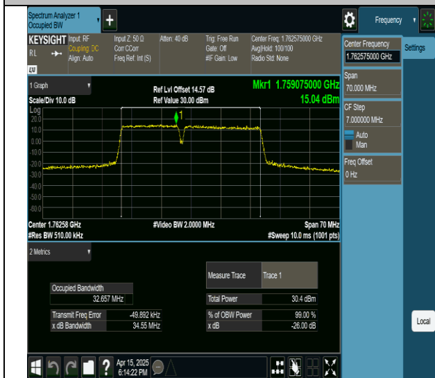
66-66-15MHz-20MHz-QPSK-QPSK-132401-132572-75RB#0-100RB#0-PASS
