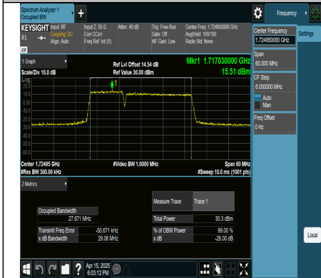
66-66-10MHz-20MHz-QPSK-QPSK-132027-132171-50RB#0-100RB#0-PASS
