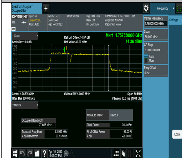
66-66-10MHz-20MHz-QPSK-QPSK-132428-132572-50RB#0-100RB#0-PASS
