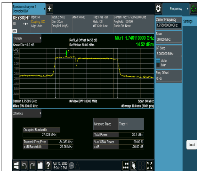
66-66-10MHz-20MHz-QPSK-QPSK-132328-132472-50RB#0-100RB#0-PASS
