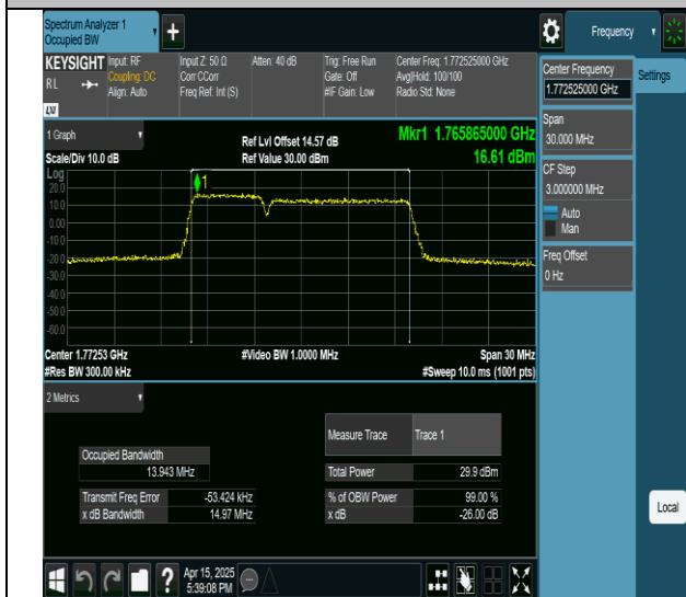
66-66-5MHz-10MHz-QPSK-QPSK-132550-132622-25RB#0-50RB#0-PASS
