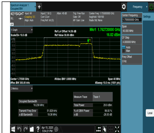
66-66-15MHz-5MHz-QPSK-QPSK-132398-132491-75RB#0-25RB#0-PASS
