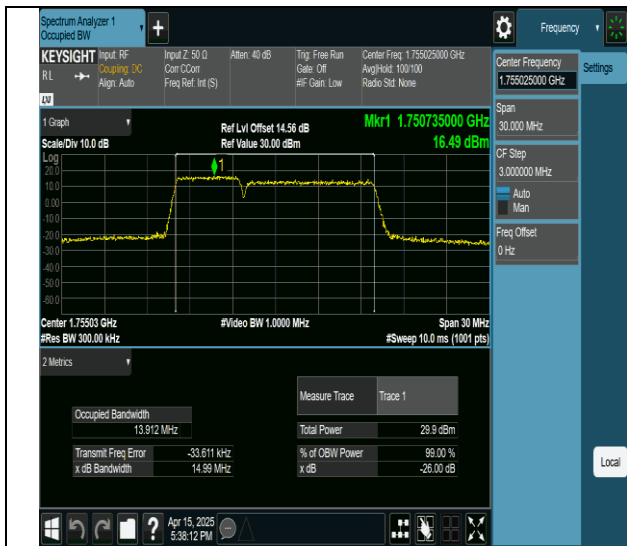
66-66-5MHz-10MHz-QPSK-QPSK-132375-132447-25RB#0-50RB#0-PASS
