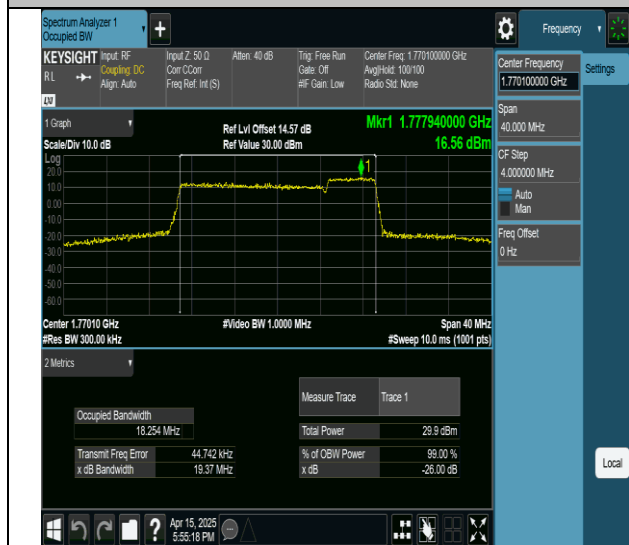
66-66-15MHz-5MHz-QPSK-QPSK-132549-132642-75RB#0-25RB#0-PASS
