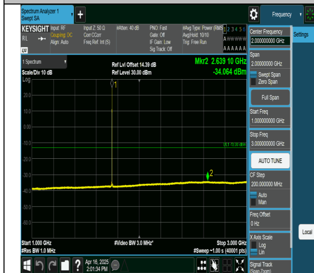
66-66-10MHz-10MHz-QPSK-QPSK-132373-132472-1RB#0- ORB#0-1000~3000MHz-PASS
