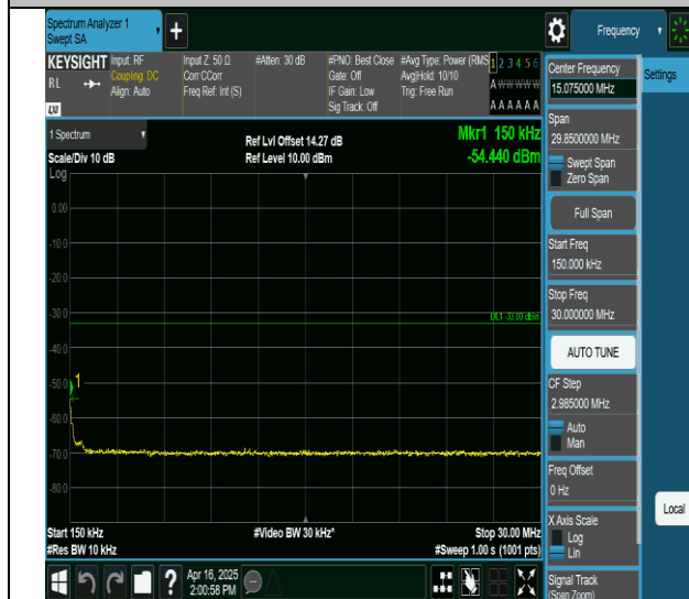
66-66-10MHz-10MHz-QPSK-QPSK-132373-132472-1RB#0- ORB#0-0.15~30MHz-PASS
