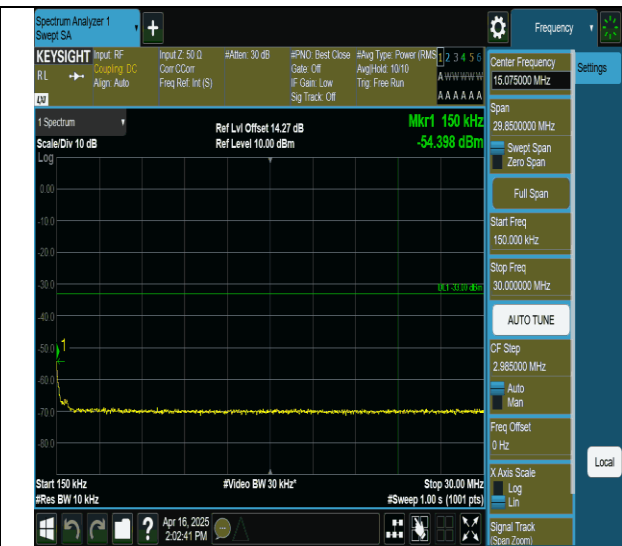
66-66-10MHz-10MHz-QPSK-QPSK-132523-132622-1RB#0- ORB#0-0.15~30MHz-PASS
