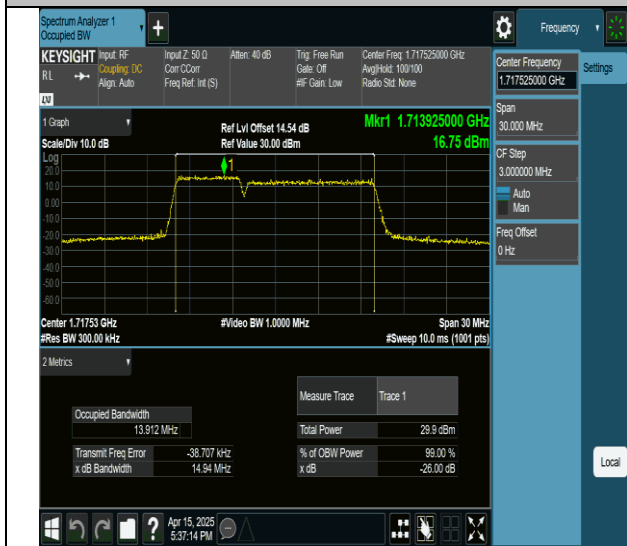
66-66-5MHz-10MHz-QPSK-QPSK-132000-132072-25RB#0-50RB#0-PASS
