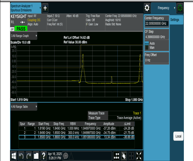
2-2-20MHz-10MHz-QPSK@QPSK-QPSK-18700-18844-1RB#0@ORB#0-1RB#49@ORB#0-PASS
