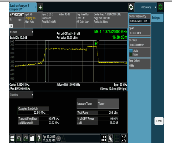
2-2-20MHz-5MHz-16QAM-16QAM-18700-18817-100RB#0-25RB#0-PASS
