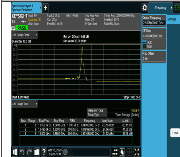
2-2-20MHz-10MHz-QPSK@QPSK-QPSK-18700-18844-1RB#0@ORB#0-ORB#0@ORB#0-PASS
