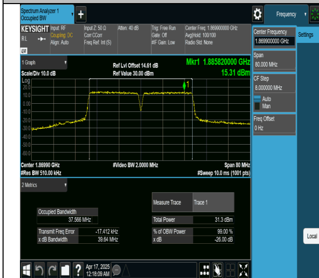
2-2-20MHz-20MHz-QPSK-QPSK-18700-18898-100RB#0-100RB#0-PASS
