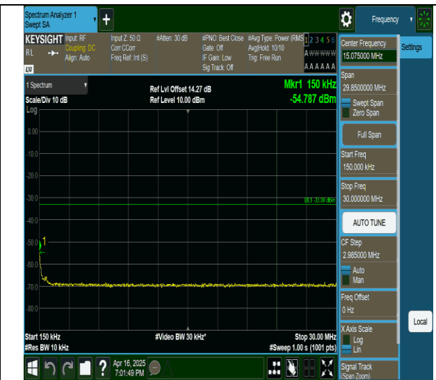
2-2-20MHz-20MHz-QPSK-QPSK-18902-19100-1RB#0-0RB#0- 0.15~30MHz-PASS
