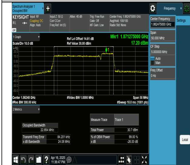
2-2-20MHz-5MHz-QPSK-QPSK-18700-18817-100RB#0-25RB#0-PASS
