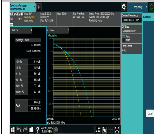
2-2-20MHz-20MHz-QPSK-QPSK-18902-19100-100RB#0-100RB#0-PASS
