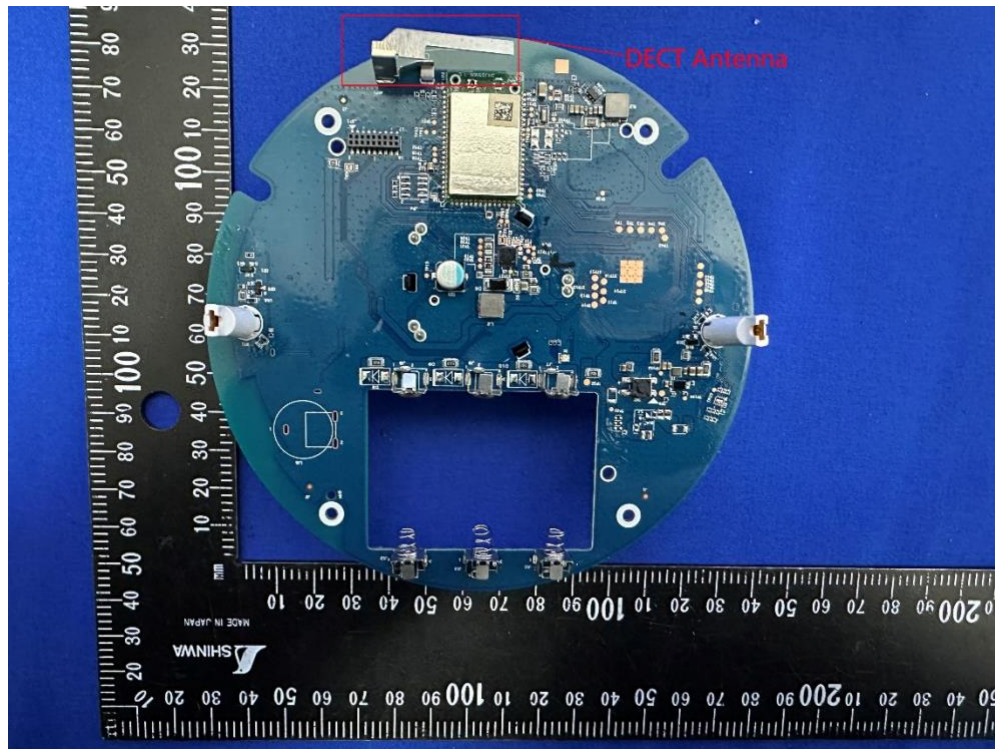
(7) EUT Photo – SSS5R0-29
