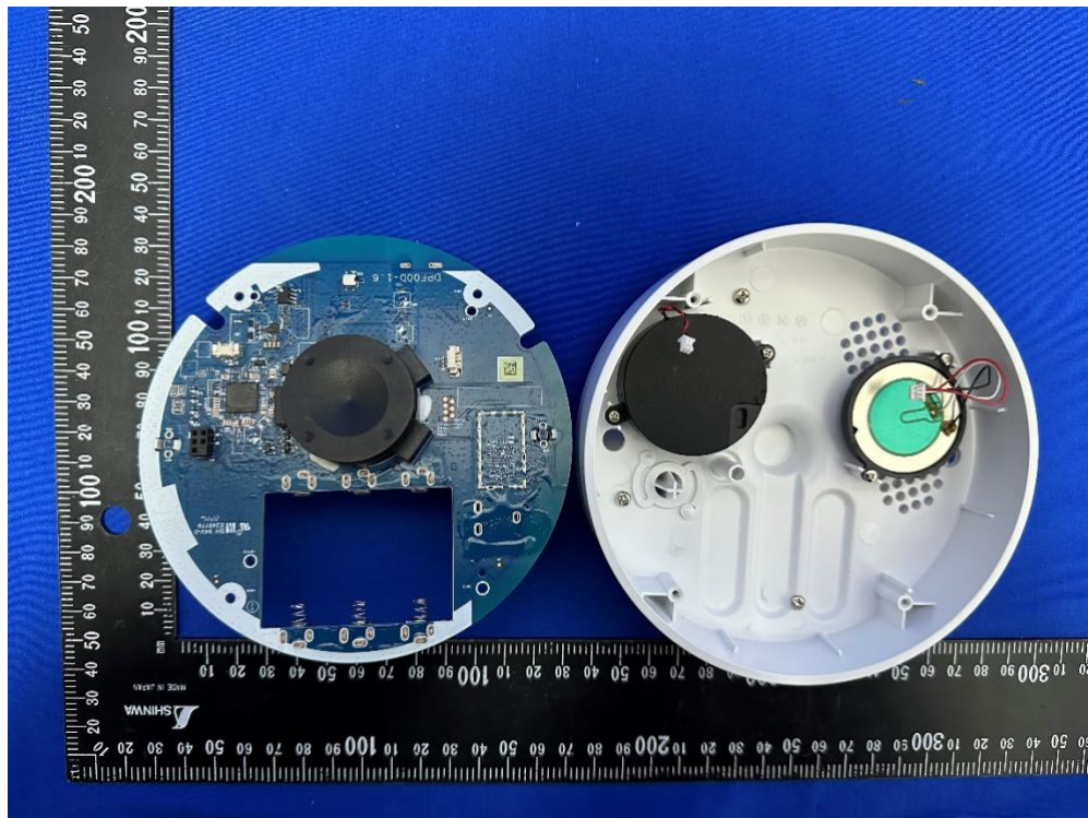
(5) EUT Photo – SSS5R0-29
