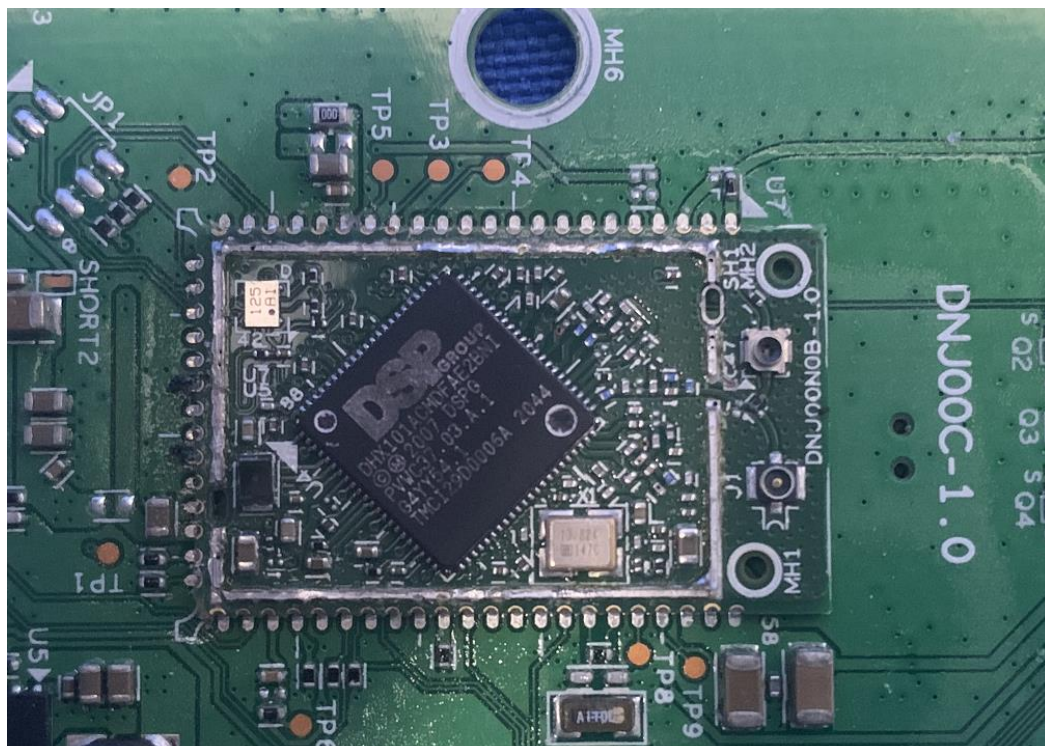
(10) EUT Photo
