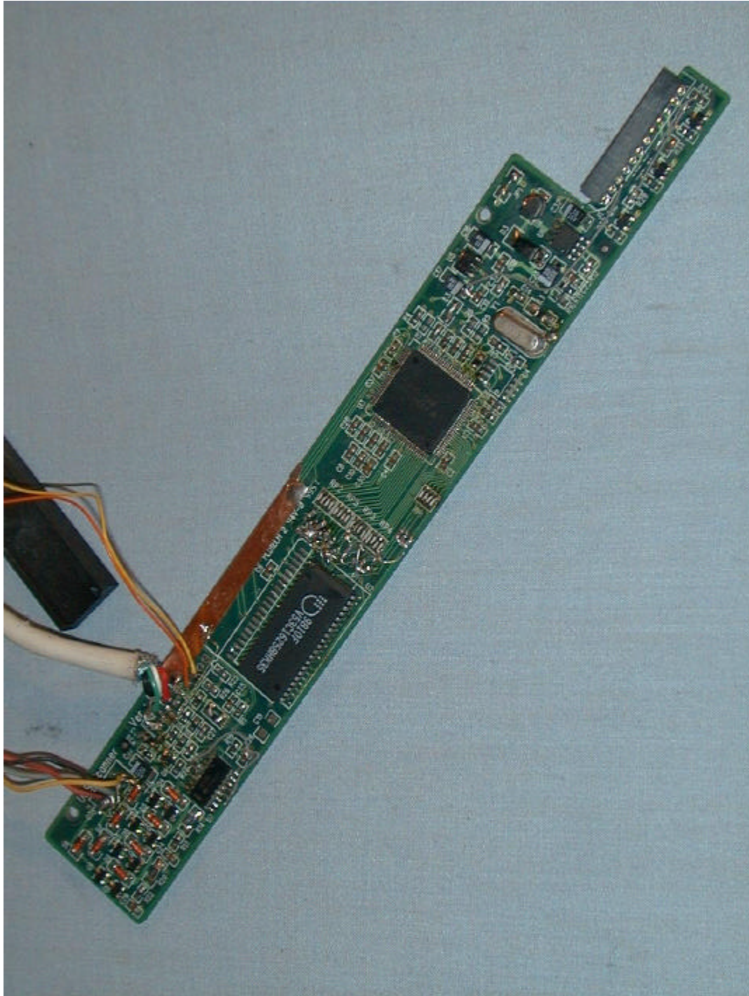
(12) EUT Photo
