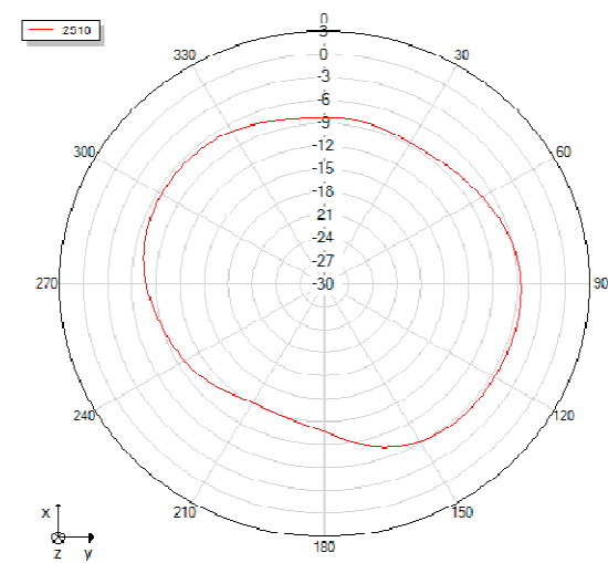
Theta=90 freq=2510MHz
