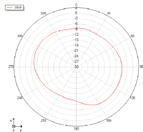
Theta=90 freq=2520MHz
