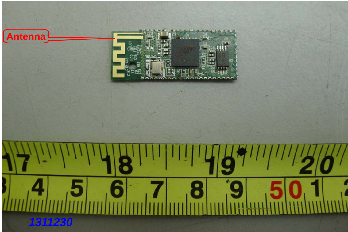
RF module
