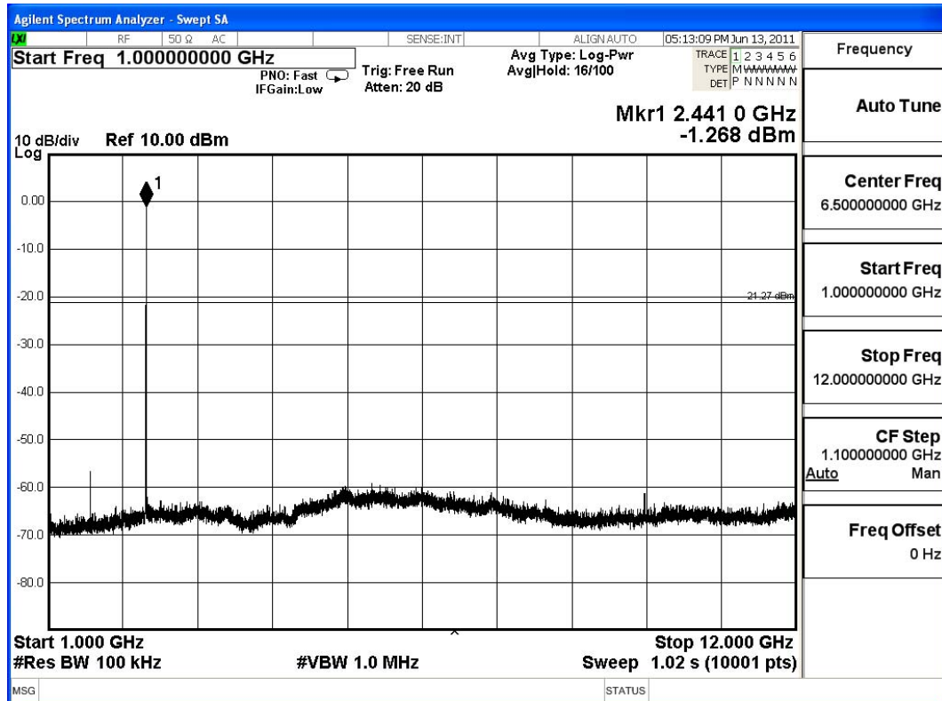
1-12GHz
