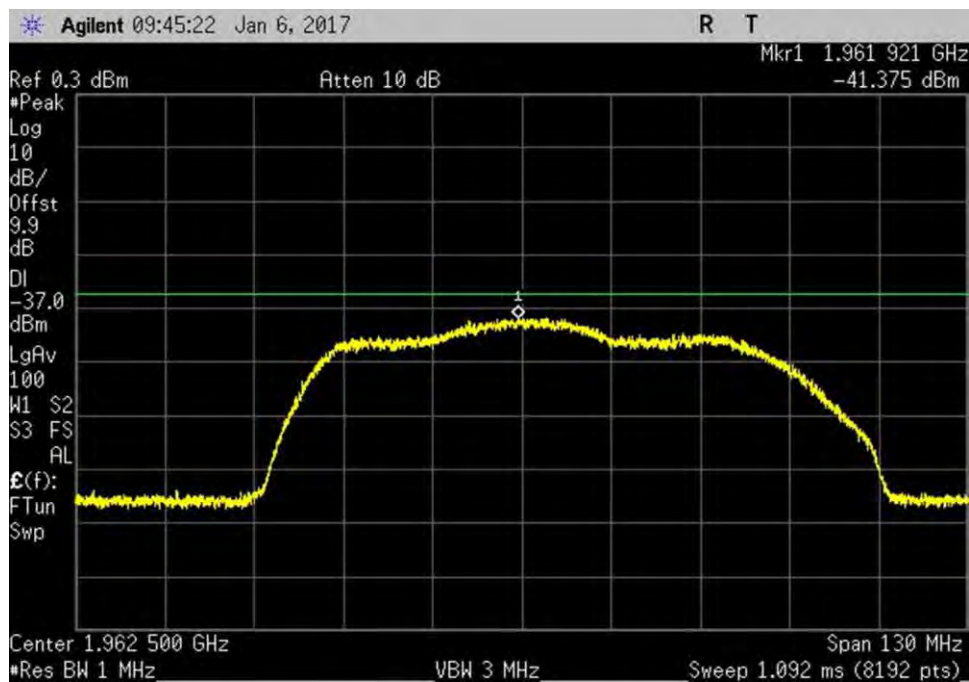
7.7.1_Noise_DL_1930-1995MHz
