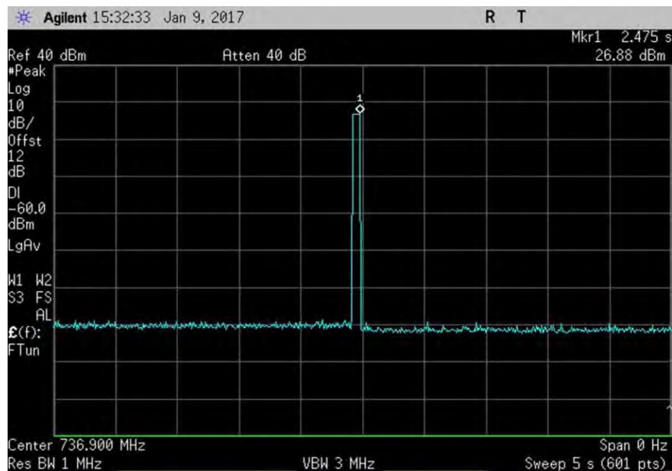
7.11.2_osc_DL_728-746MHzPk
