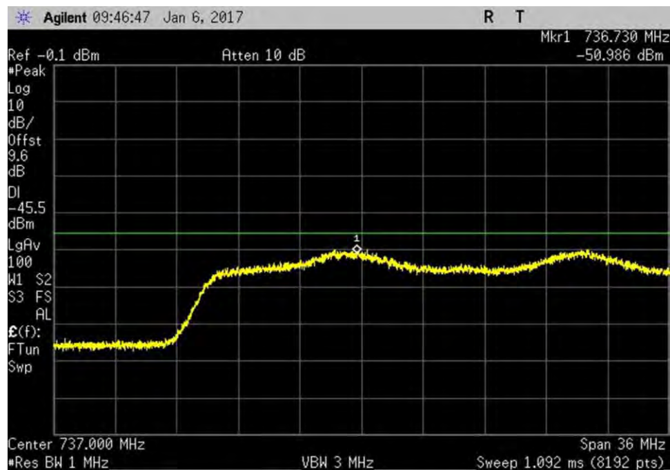
7.7.1_Noise_DL_728-746MHz
