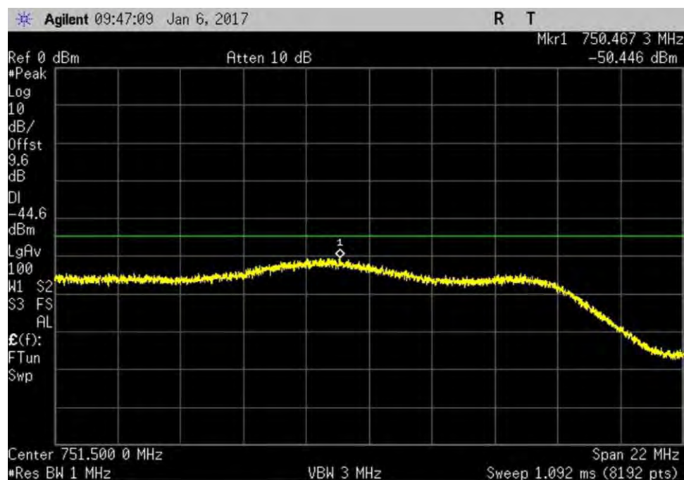
7.7.1_Noise_DL_746-757MHz
