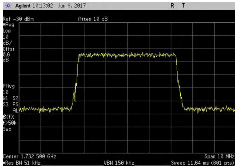
7.10_OBW_UL_1710-1755MHz_LTE_In
