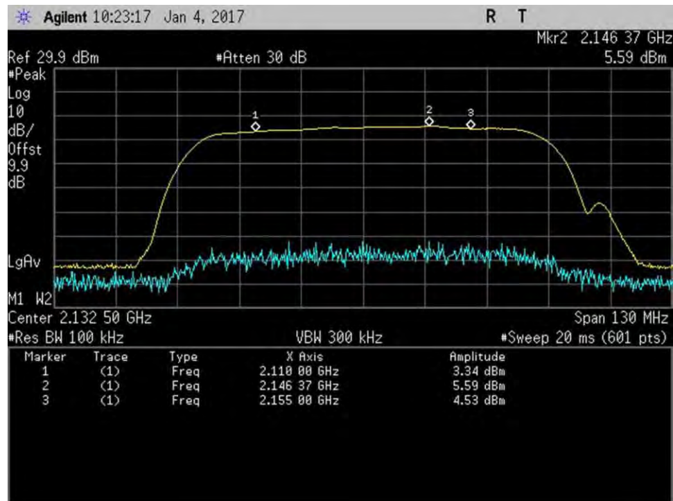
7.1_Band Verify_DL_2110-2155MHz_Zoom
