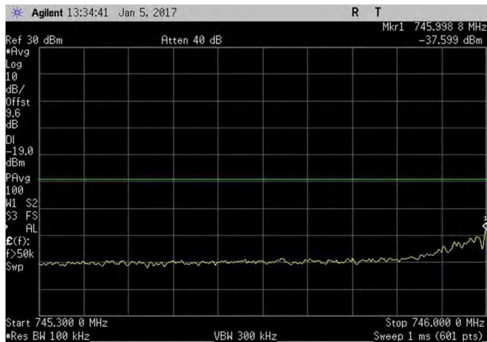
7.5_OBE_DL_746-757MHz_L_PreAGC_LTE
