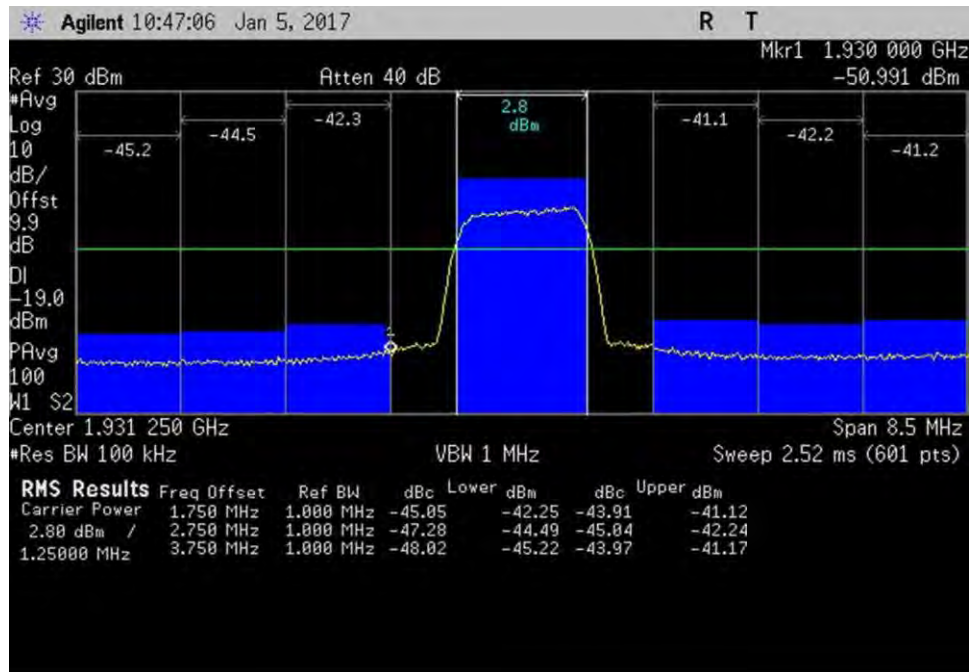
7.5_OBE_DL_1930-1995MHz_L_PreAGC_CDMA
