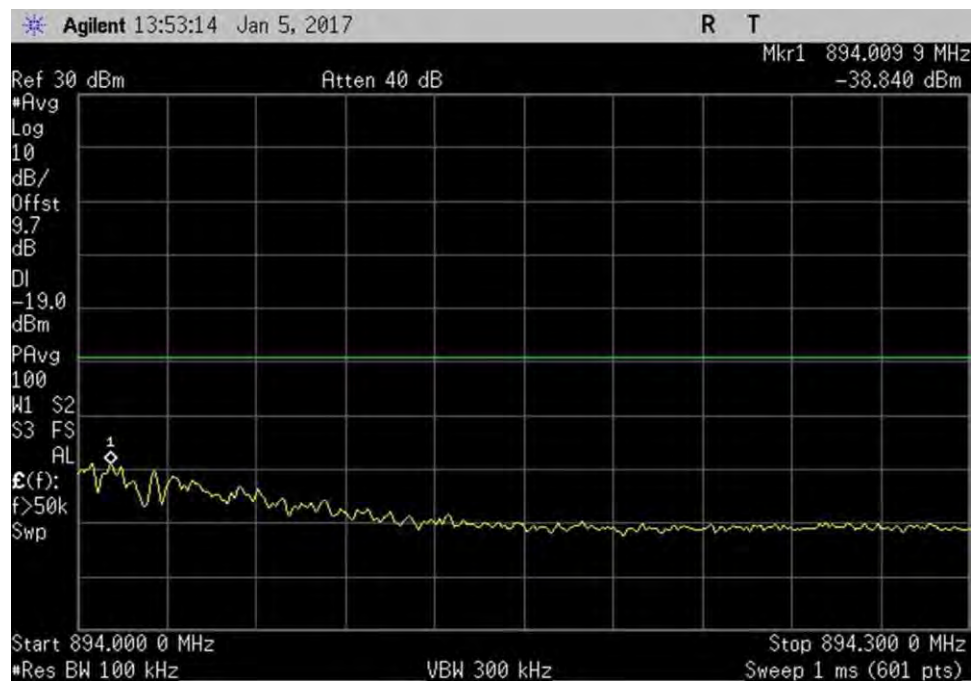
7.5_OBE_DL_869-894MHz_H_PreAGC_LTE
