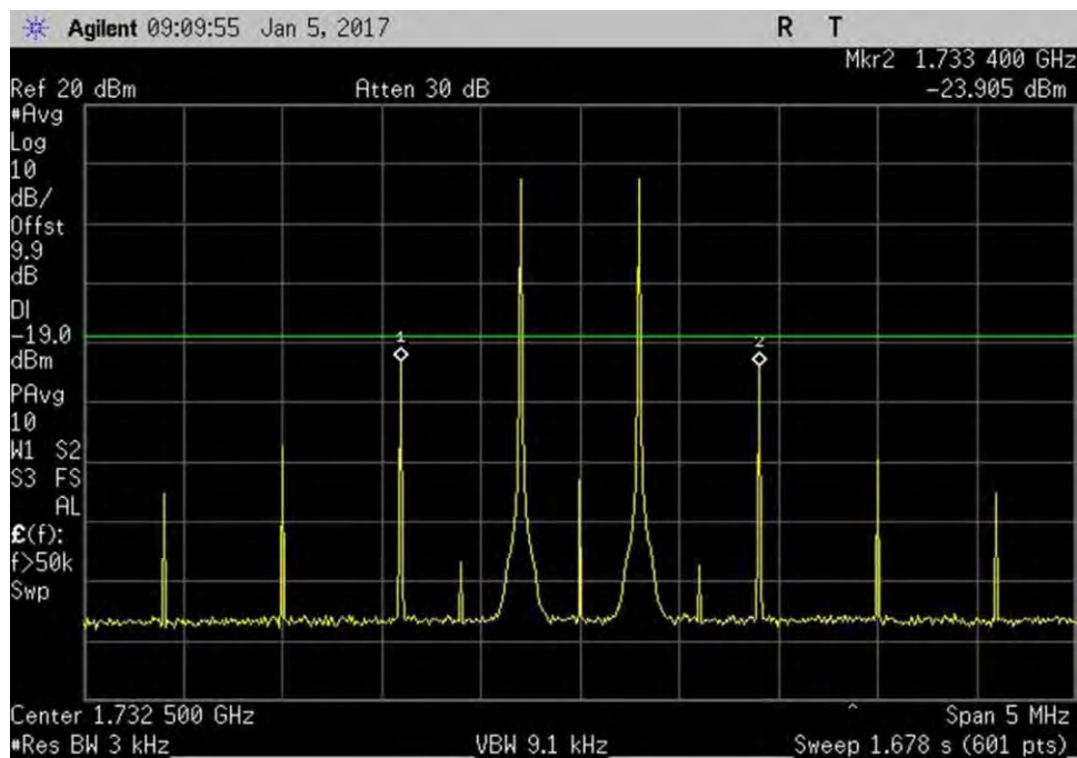
7.4_Intermod_UL_1710-1755MHz
