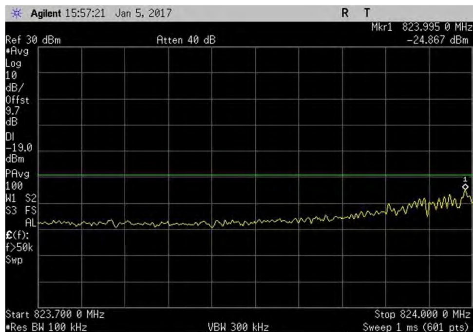
7.5_OBE_UL_824-849MHz_L_PreAGC_LTE
