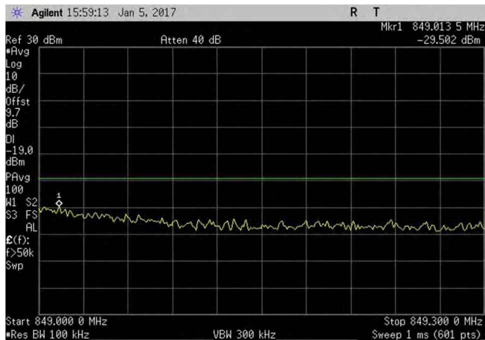
7.5_OBE_UL_824-849MHz_H_PreAGC_LTE
