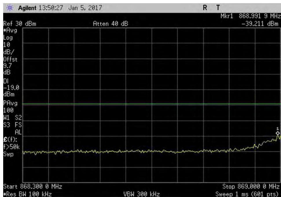
7.5_OBE_DL_869-894MHz_L_PreAGC_LTE
