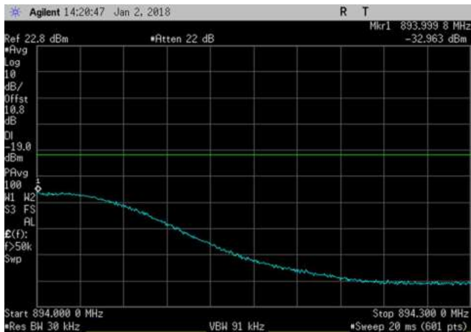
DL_ 894- 894.3MHz_GSM
