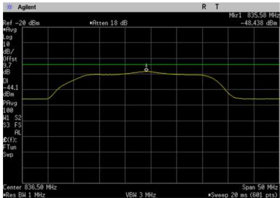
UL_824-849MHz
