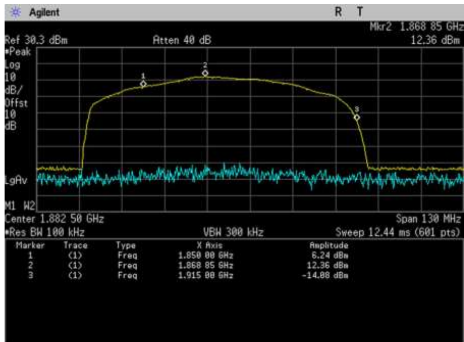
UL_1850-1915MHz
