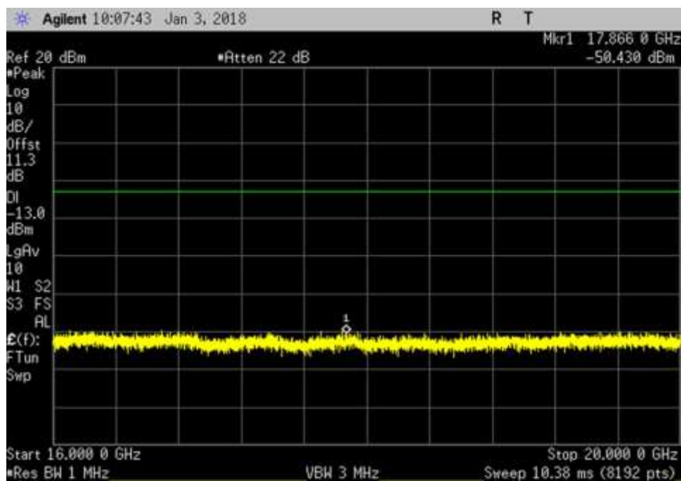
UL_ 16000- 20000MHz_AWGN
