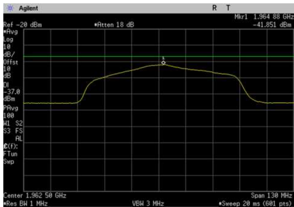
DL_1930-1995MHz
