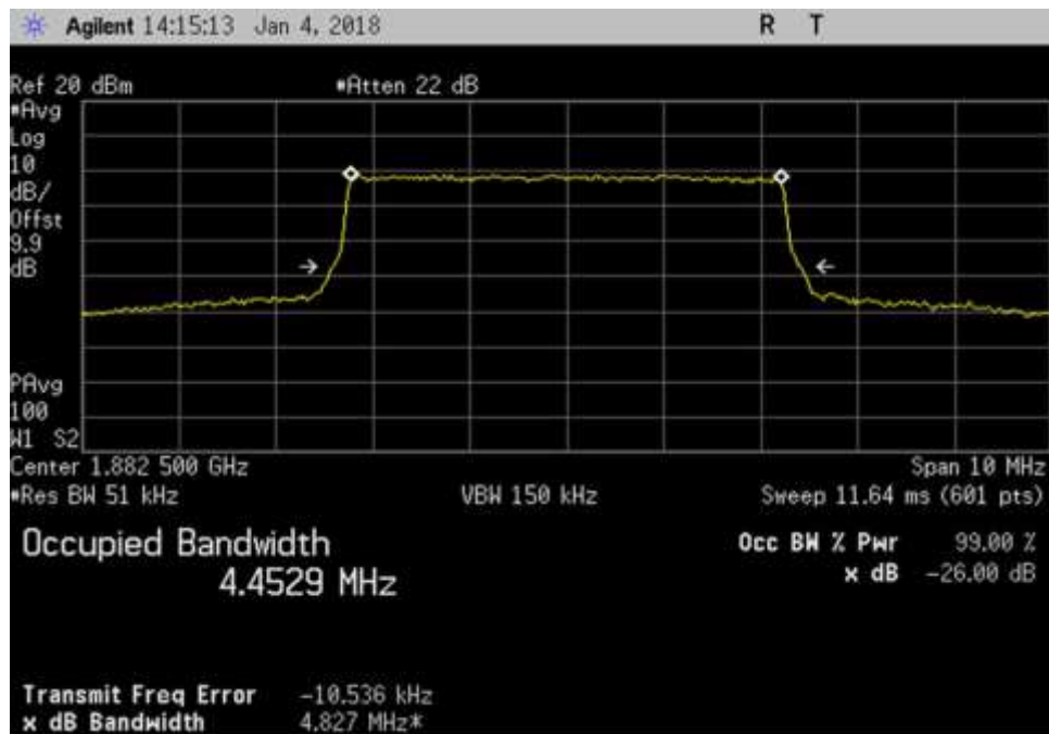
UL_ 1882.5MHz_LTE
