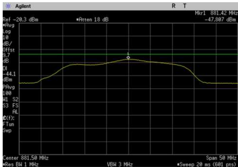
DL_869-894MHz
