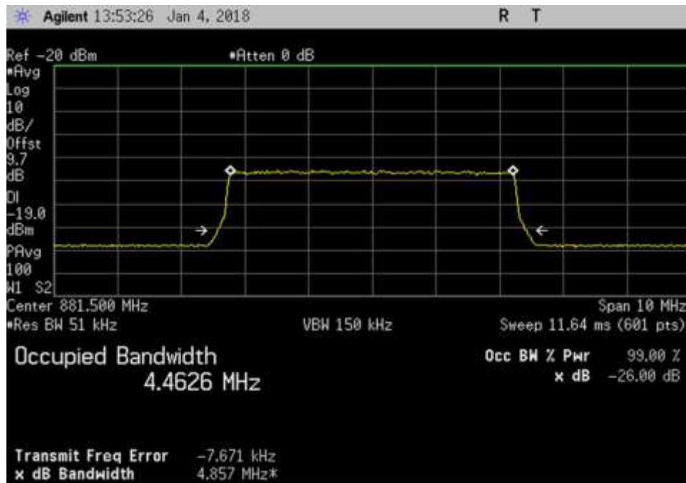
DL_881.5MHz_LTE
