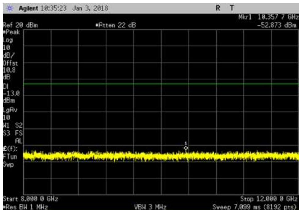
DL_ 8000- 12000MHz_AWGN
