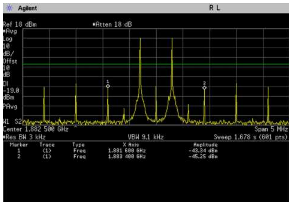
UL_1850-1915MHz_+10dB
