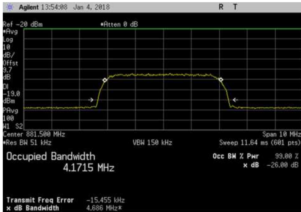
DL_881.5MHz_WCDMA
