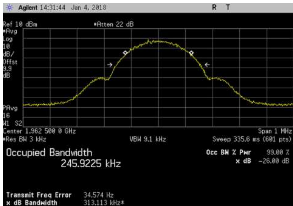
DL_1962.5MHz_GSM
