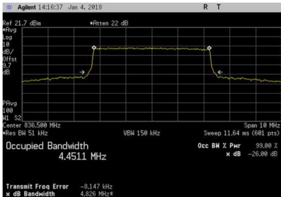
UL_ 836.5MHz_LTE
