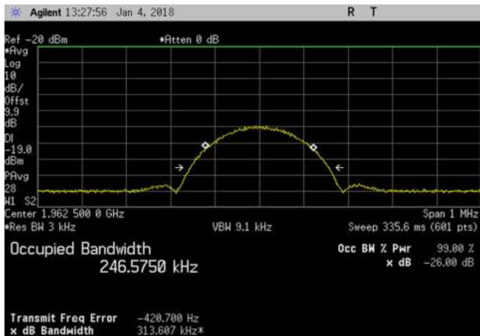
DL_1962.5MHz_EDGE
