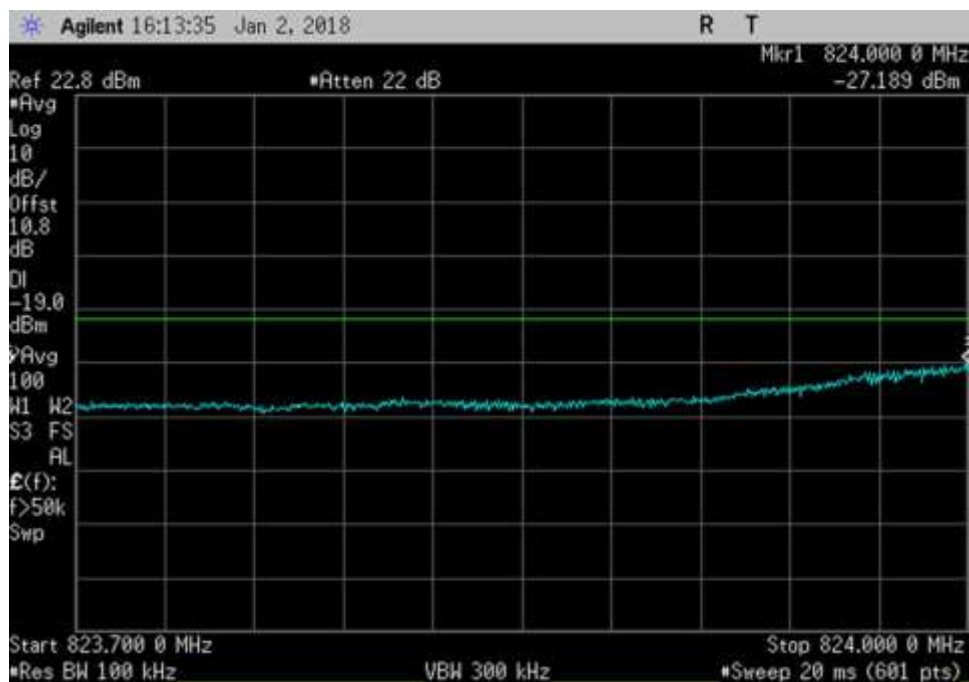
UL_ 823.7- 824MHz_LTE
