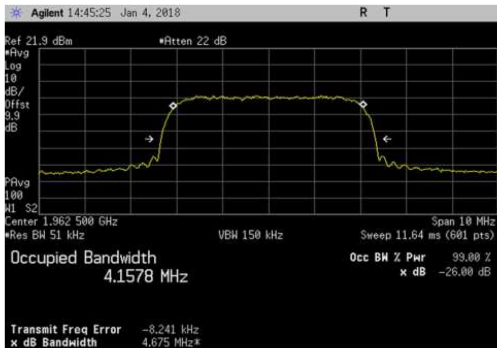
DL_1962.5MHz_WCDMA
