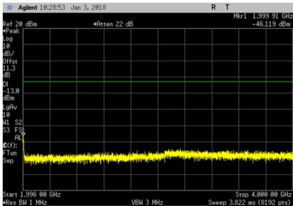
DL_1996-4000MHz_AWGN
