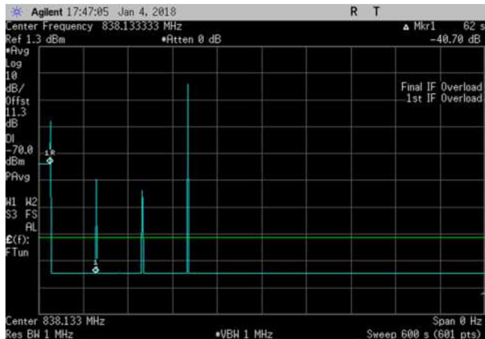
UL_ 838.133333MHz_600sec
