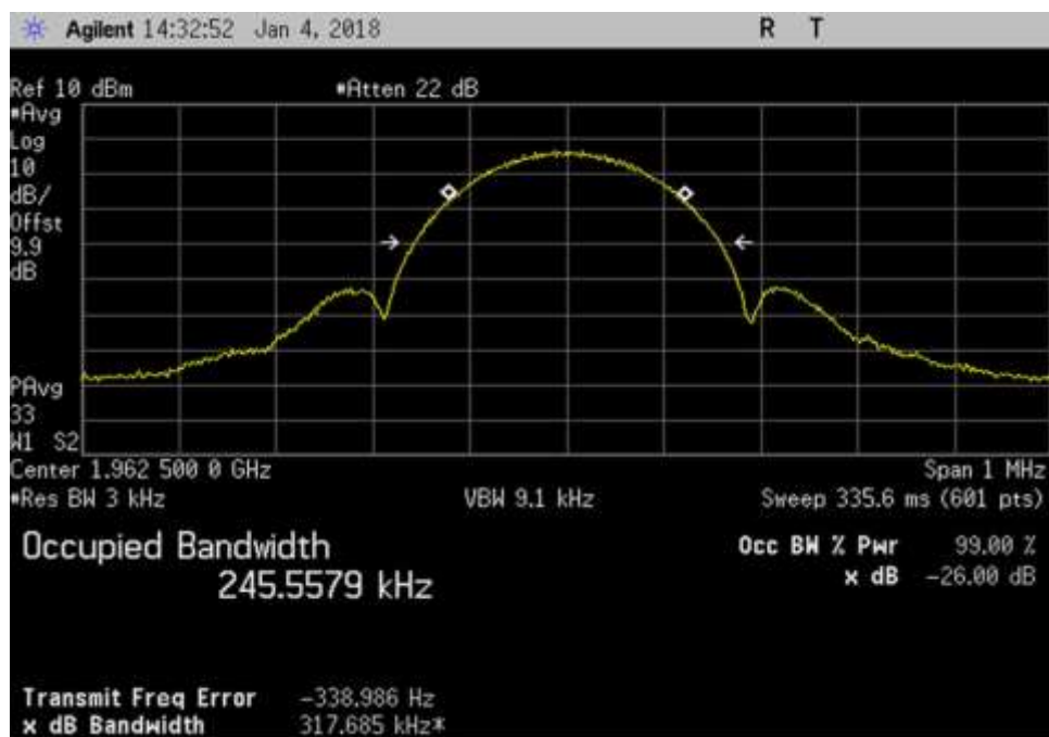
DL_1962.5MHz_EDGE
