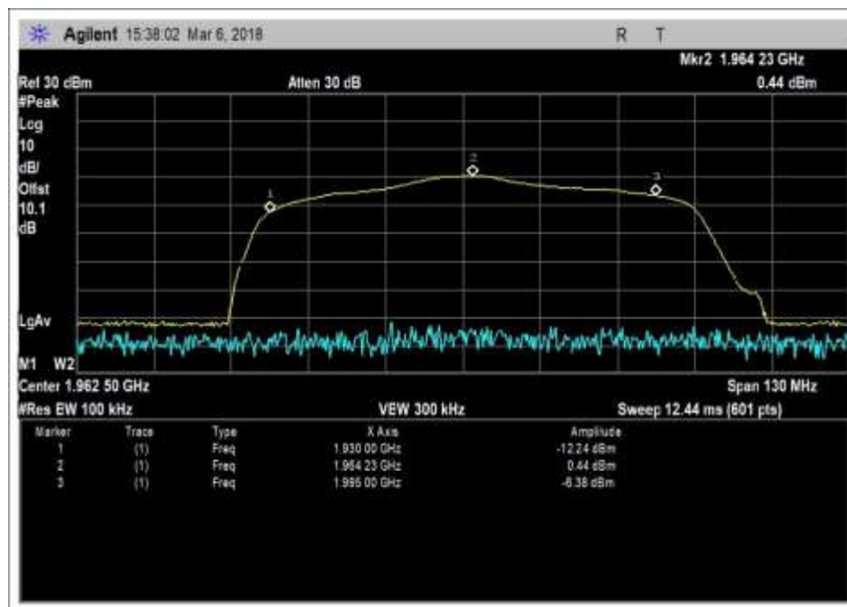
DL_1930-1995MHz
