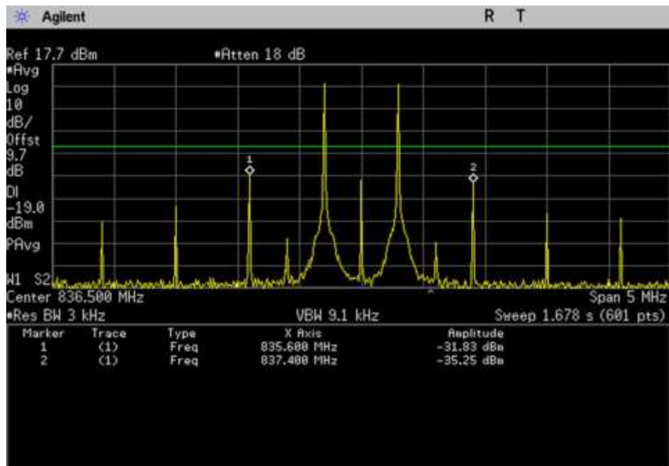
UL_824-849MHz_+10dB
