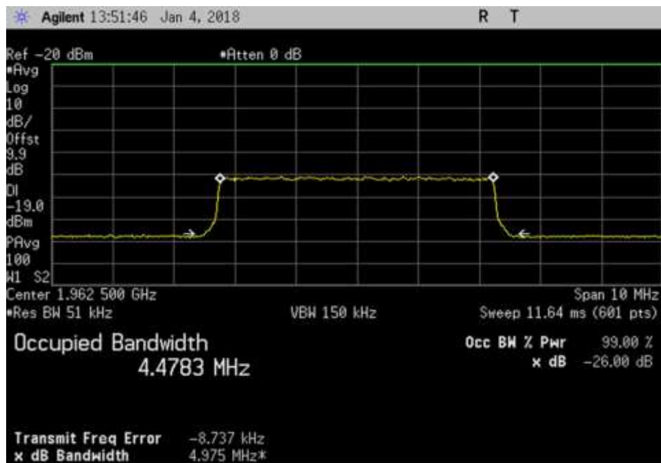
DL_1962.5MHz_LTE
