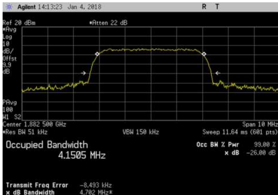
UL_ 1882.5MHz_WCDMA
