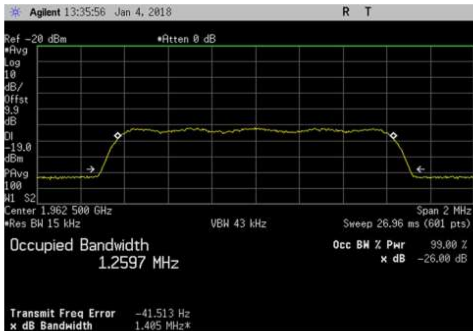
DL_1962.5MHz_CDMA
