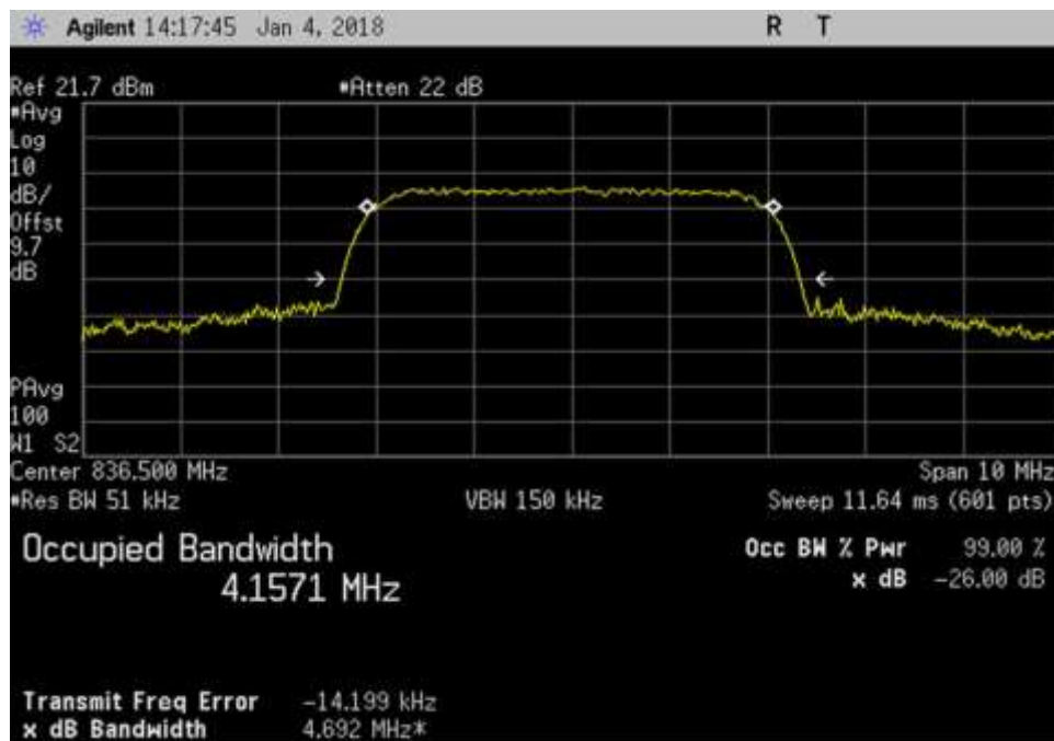
UL_ 836.5MHz_WCDMA
