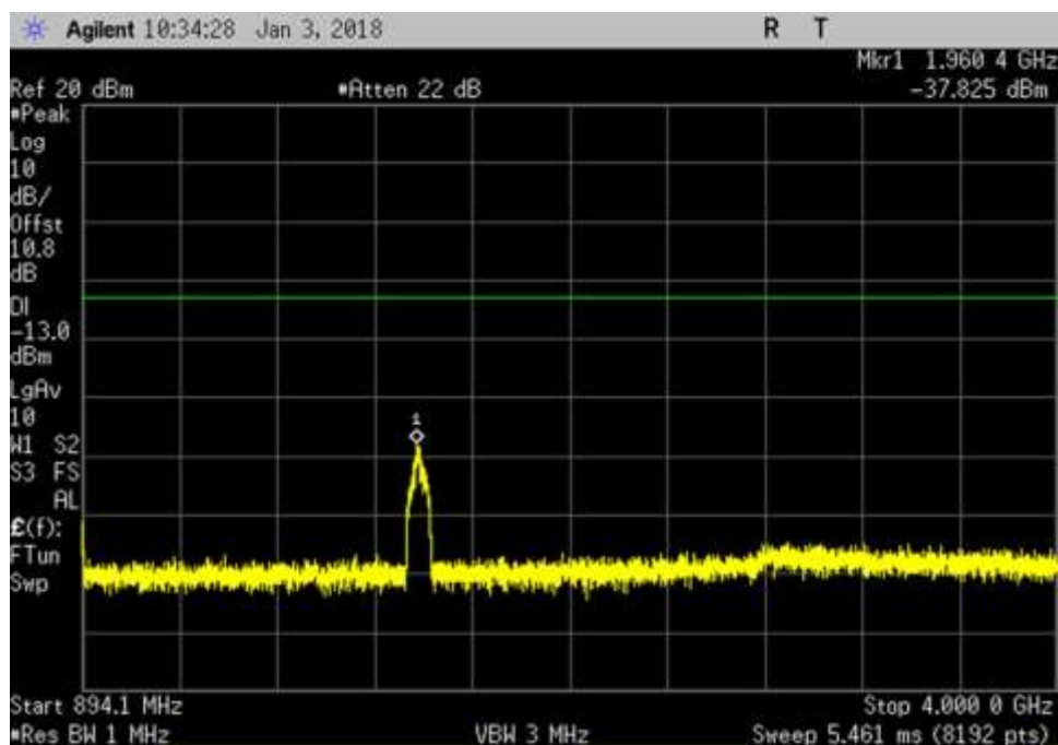
DL_ 894.1- 4000MHz_AWGN
