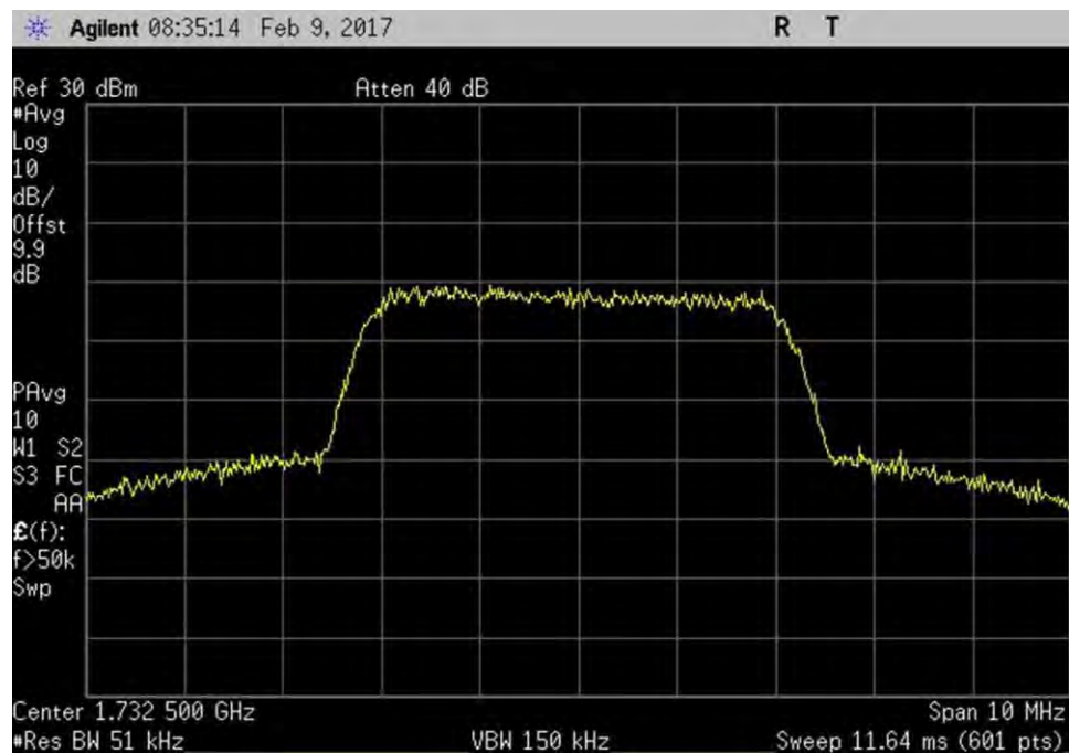
7.10_OBW_UL_1710-1755MHz_WCDMA_Out
