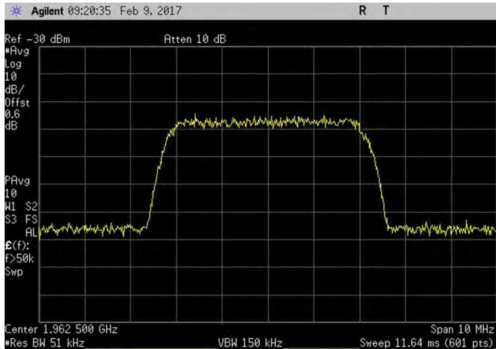
7.10_OBW_DL_1930-1995MHz_WCDMA_In
