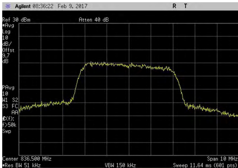
7.10_OBW_UL_824-849MHz_WCDMA_Out
