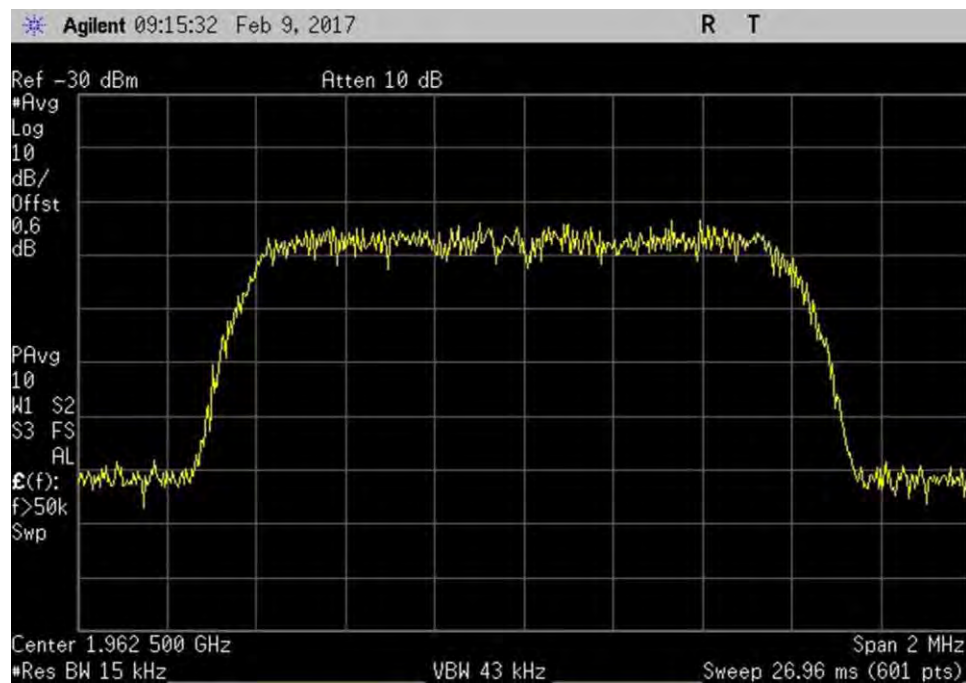
7.10_OBW_DL_1930-1995MHz_CDMA_In
