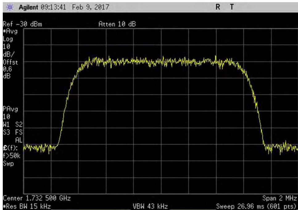
7.10_OBW_UL_1710-1755MHz_CDMA_In
