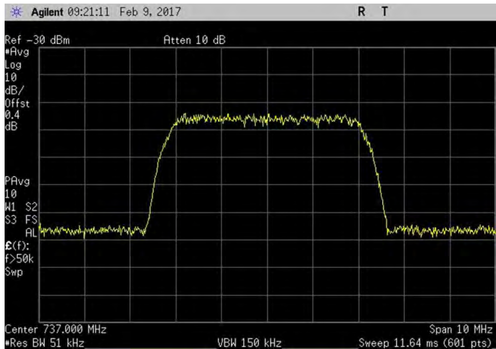
7.10_OBW_DL_728-746MHz_WCDMA_In
