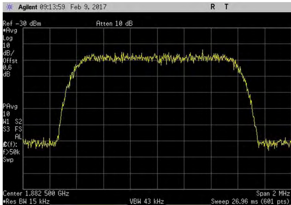
7.10_OBW_UL_1850-1915MHz_CDMA_In
