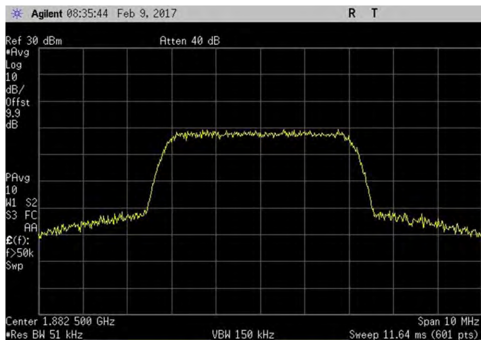
7.10_OBW_UL_1850-1915MHz_WCDMA_Out
