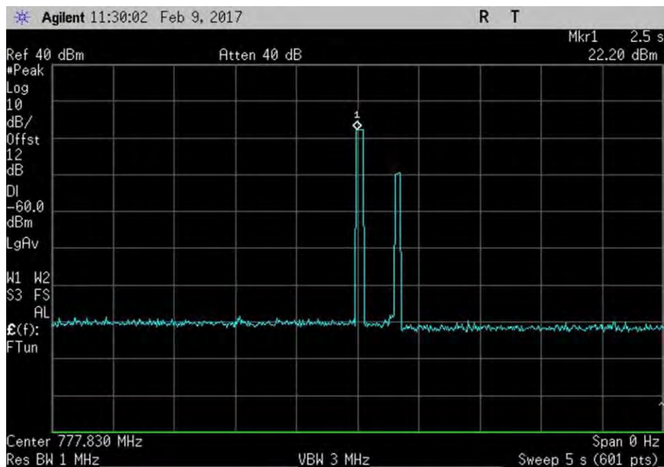
7.11.2_osc_UL_776-787MHzPk
