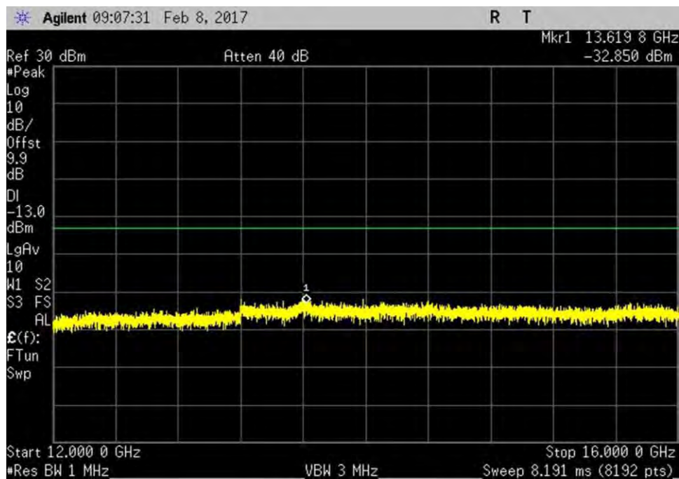
7.6_CSE_DL_1930-1995MHz_R4
