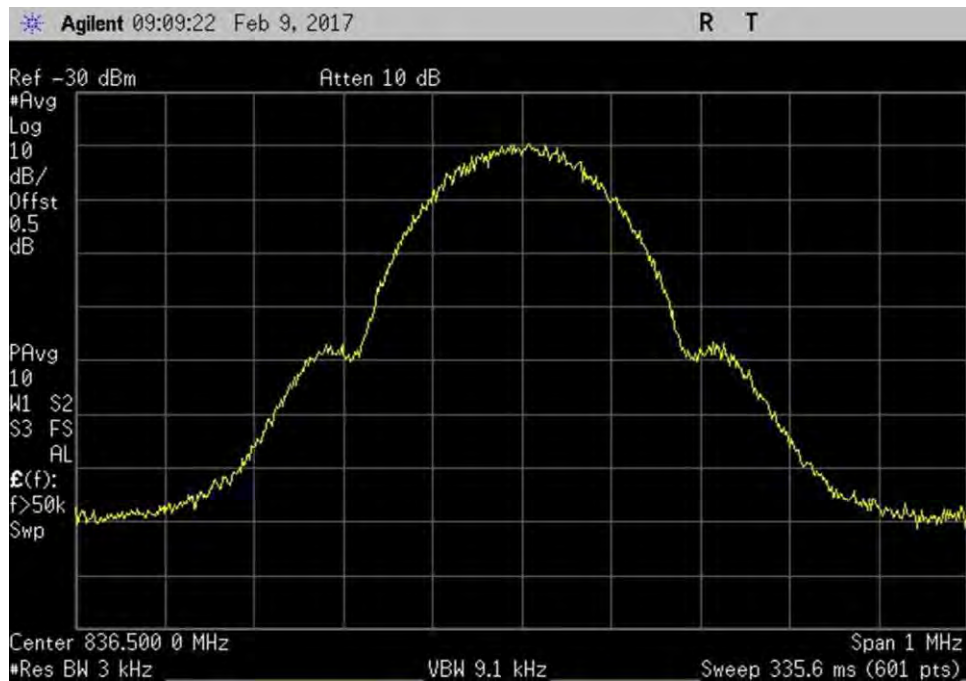
7.10_OBW_UL_824-849MHz_GSM_In
