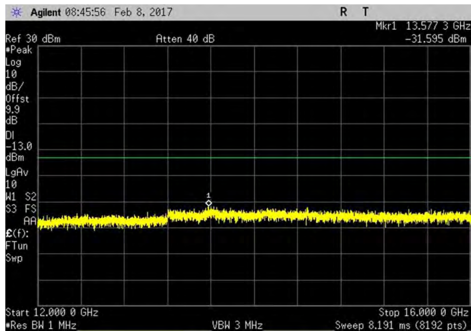
7.6_CSE_UL_1710-1755MHz_R4
