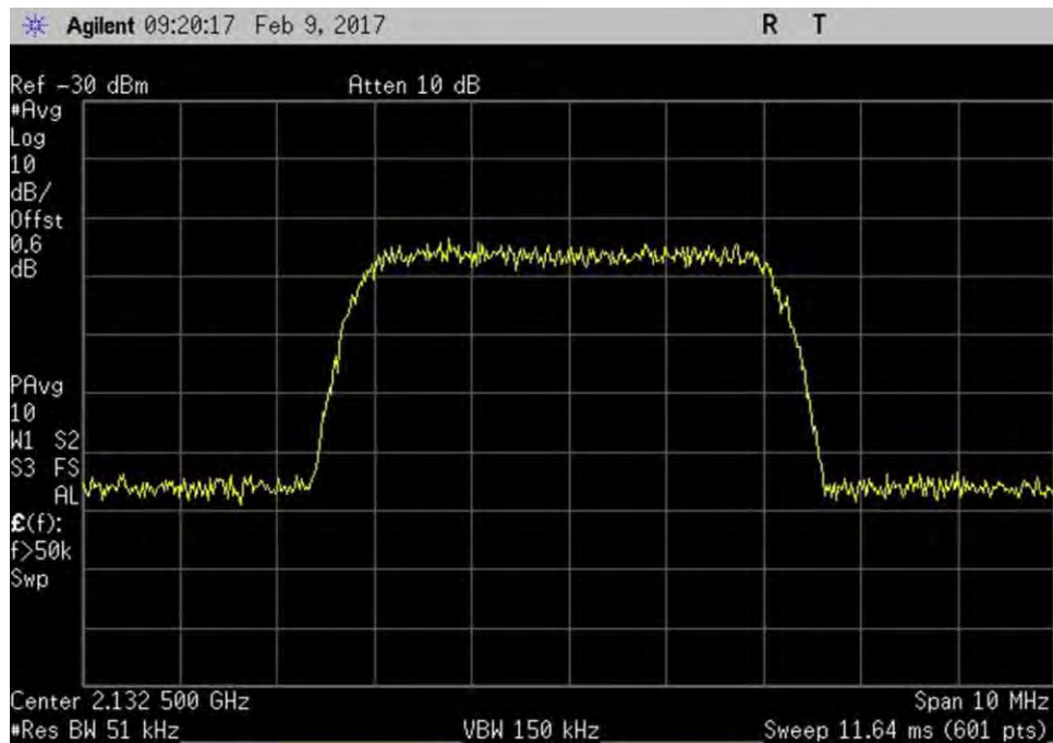
7.10_OBW_DL_2110-2155MHz_WCDMA_In
