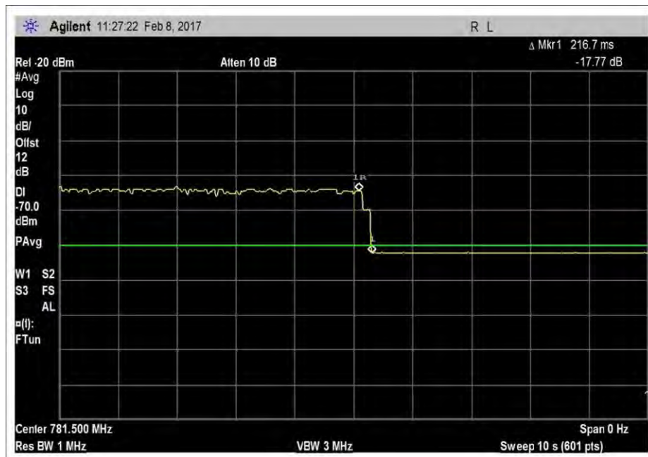
7.7.2_VarNoise_UL_776-787MHz
