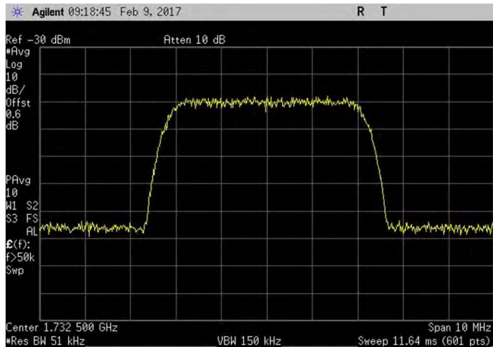
7.10_OBW_UL_1710-1755MHz_WCDMA_In
