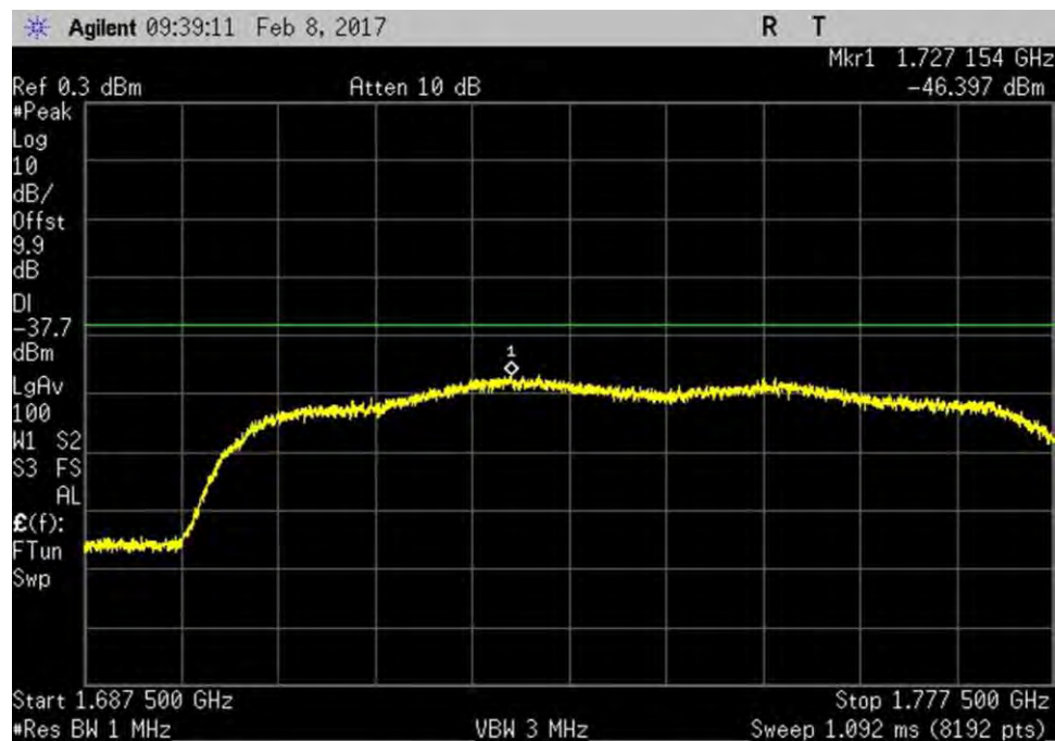
7.7.1_Noise_UL_1710-1755MHz
