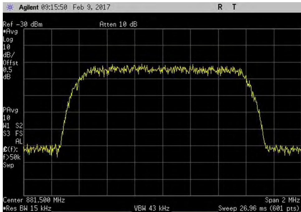
7.10_OBW_DL_869-894MHz_CDMA_In
