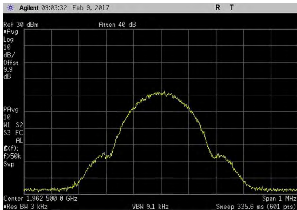
7.10_OBW_DL_1930-1995MHz_GSM_Out
