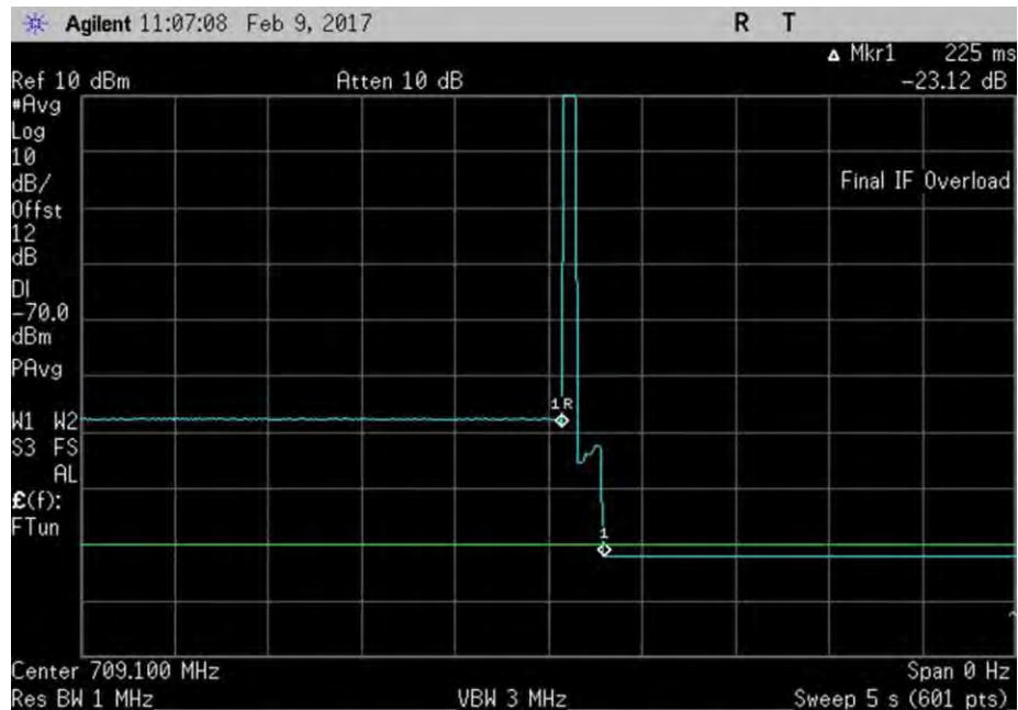
7.11.2_osc_UL_698-716MHz
