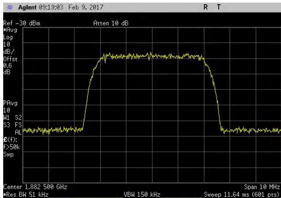
7.10_OBW_UL_1850-1915MHz_WCDMA_In
