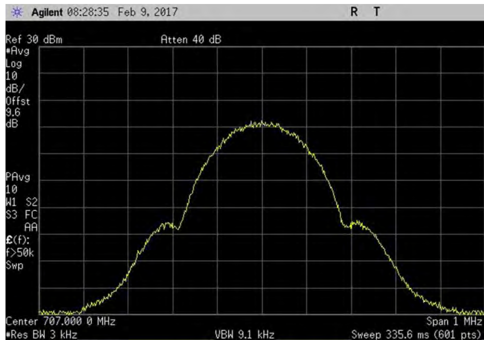
7.10_OBW_UL_698-716MHz_GSM_Out
