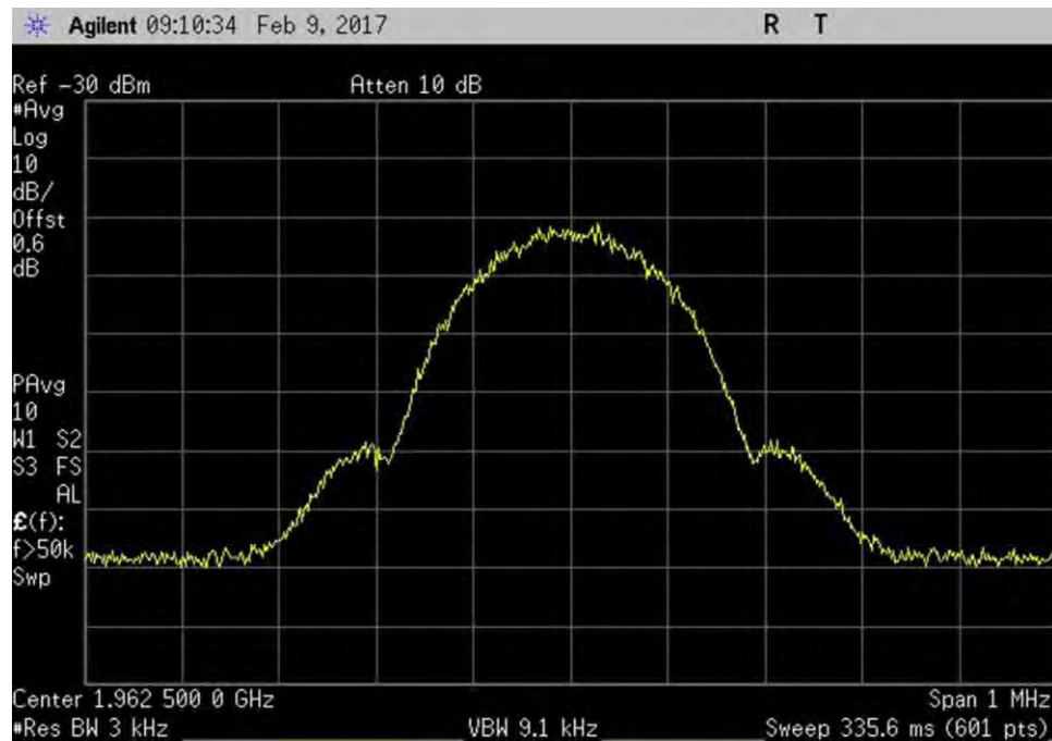
7.10_OBW_DL_1930-1995MHz_GSM_In
