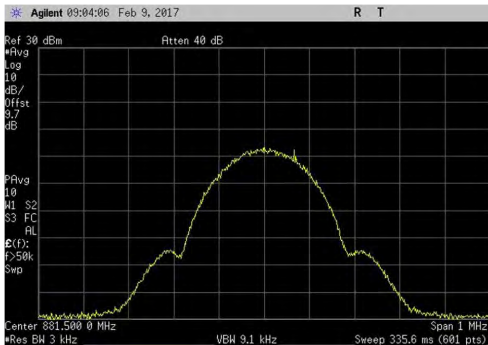
7.10_OBW_DL_869-894MHz_GSM_Out
