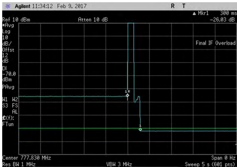
7.11.2_osc_UL_776-787MHz
