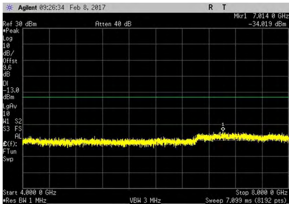
7.6_CSE_DL_728-746MHz_R2
