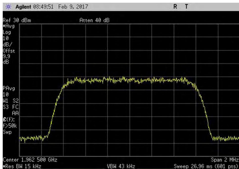
7.10_OBW_DL_1930-1995MHz_CDMA_Out
