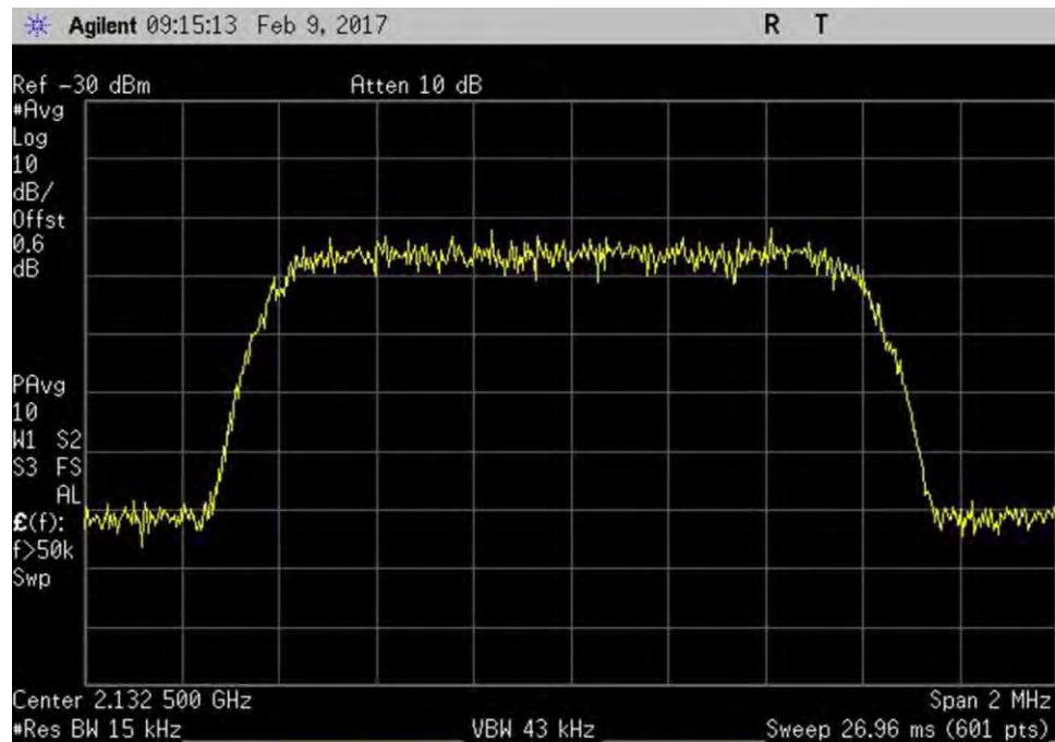
7.10_OBW_DL_2110-2155MHz_CDMA_In
