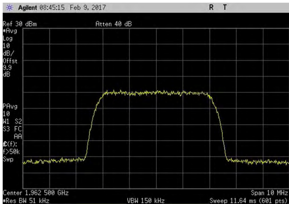
7.10_OBW_DL_1930-1995MHz_WCDMA_Out
