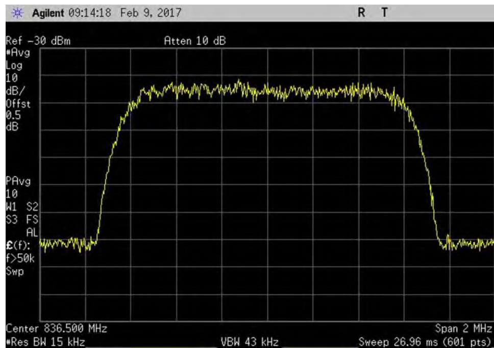
7.10_OBW_UL_824-849MHz_CDMA_In
