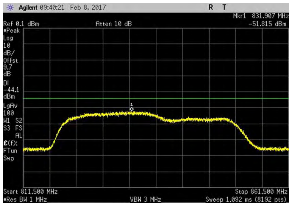
7.7.1_Noise_UL_824-849MHz
