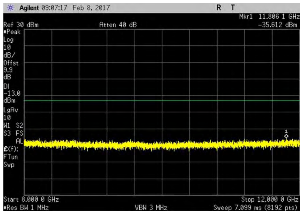
7.6_CSE_DL_1930-1995MHz_R3
