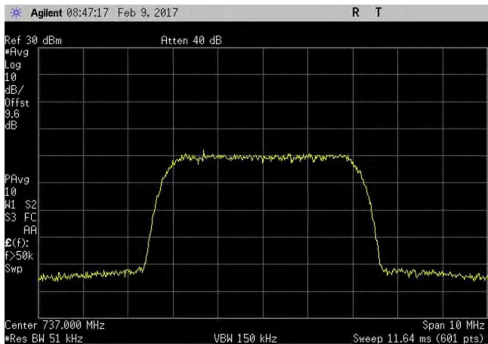
7.10_OBW_DL_728-746MHz_WCDMA_Out
