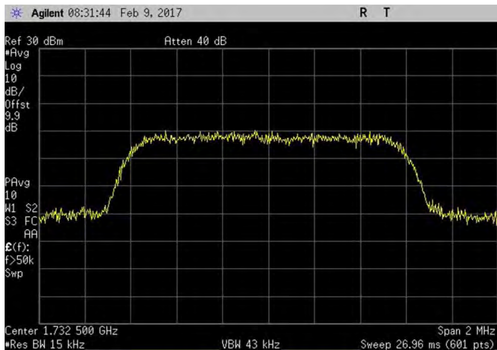
7.10_OBW_UL_1710-1755MHz_CDMA_Out
