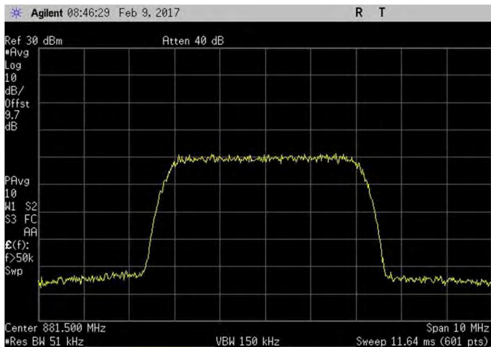
7.10_OBW_DL_869-894MHz_WCDMA_Out
