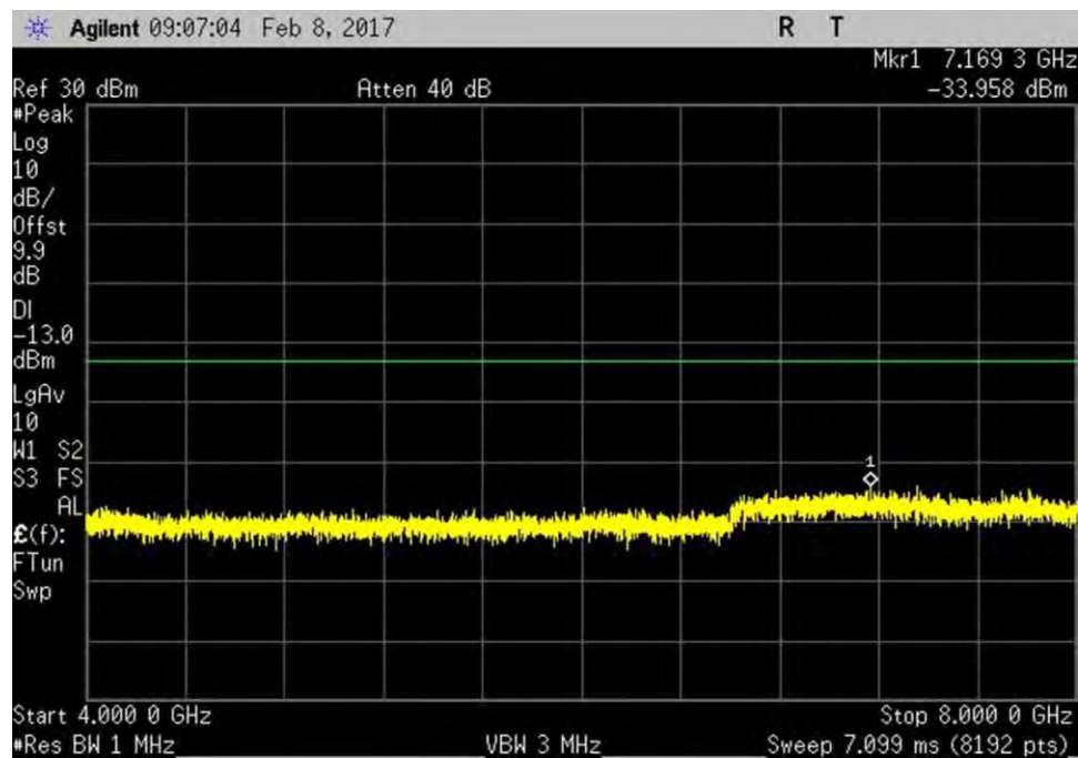
7.6_CSE_DL_1930-1995MHz_R2
