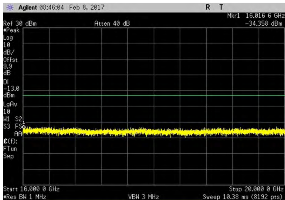
7.6_CSE_UL_1710-1755MHz_R5
