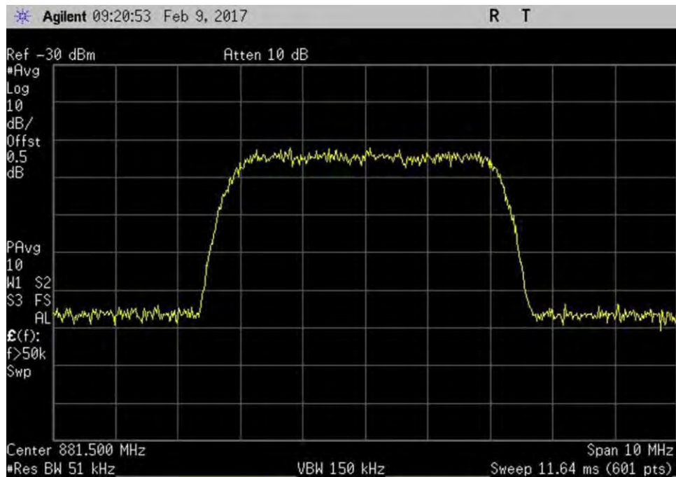
7.10_OBW_DL_869-894MHz_WCDMA_In
