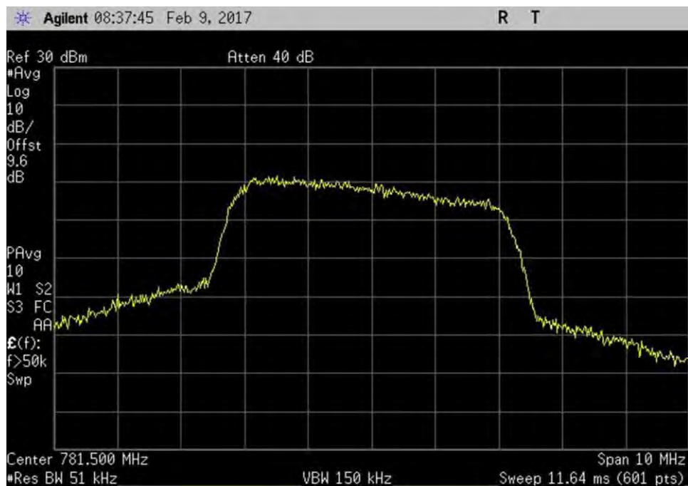
7.10_OBW_UL_776-787MHz_WCDMA_Out
