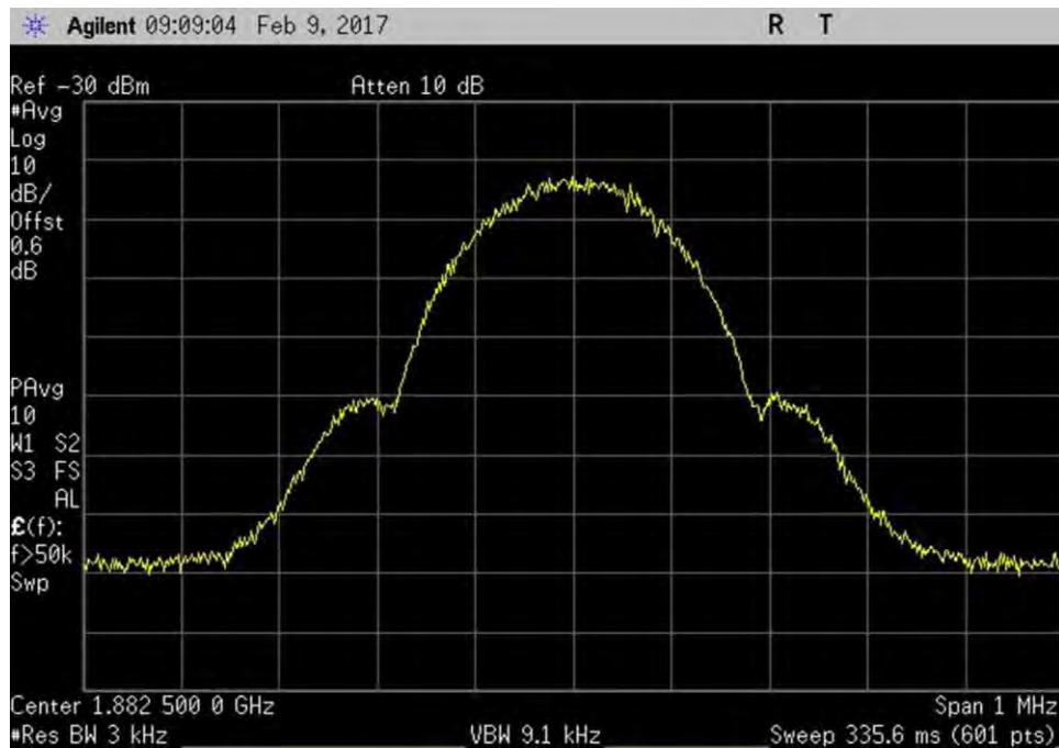
7.10_OBW_UL_1850-1915MHz_GSM_In
