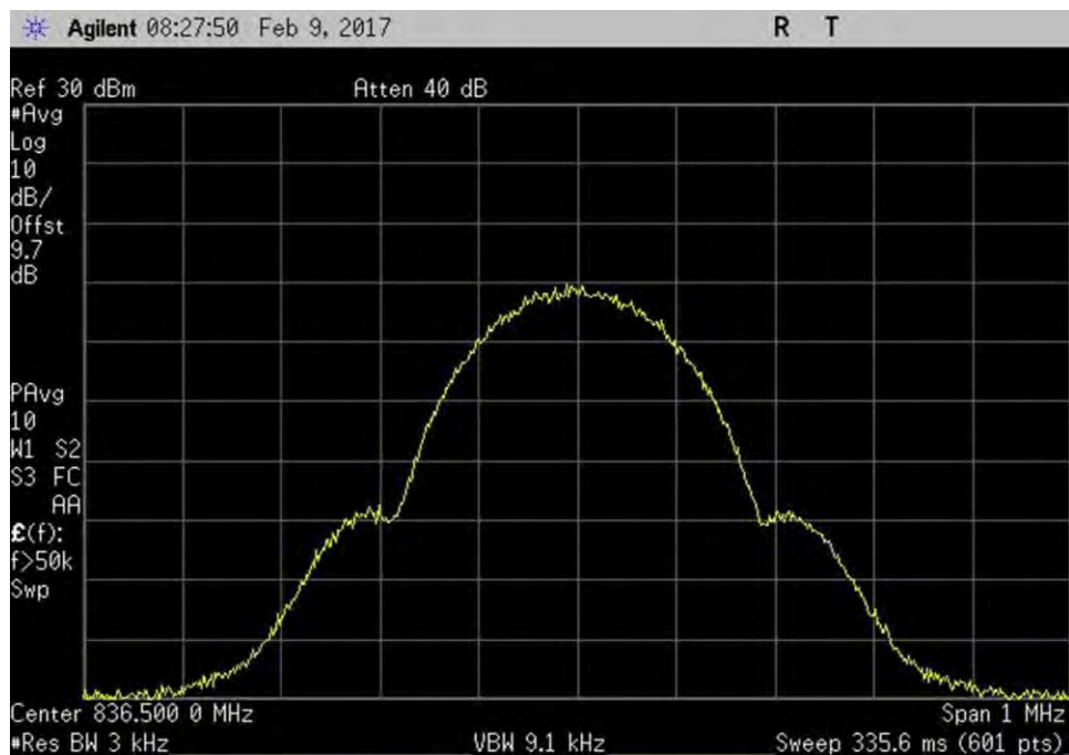
7.10_OBW_UL_824-849MHz_GSM_Out
