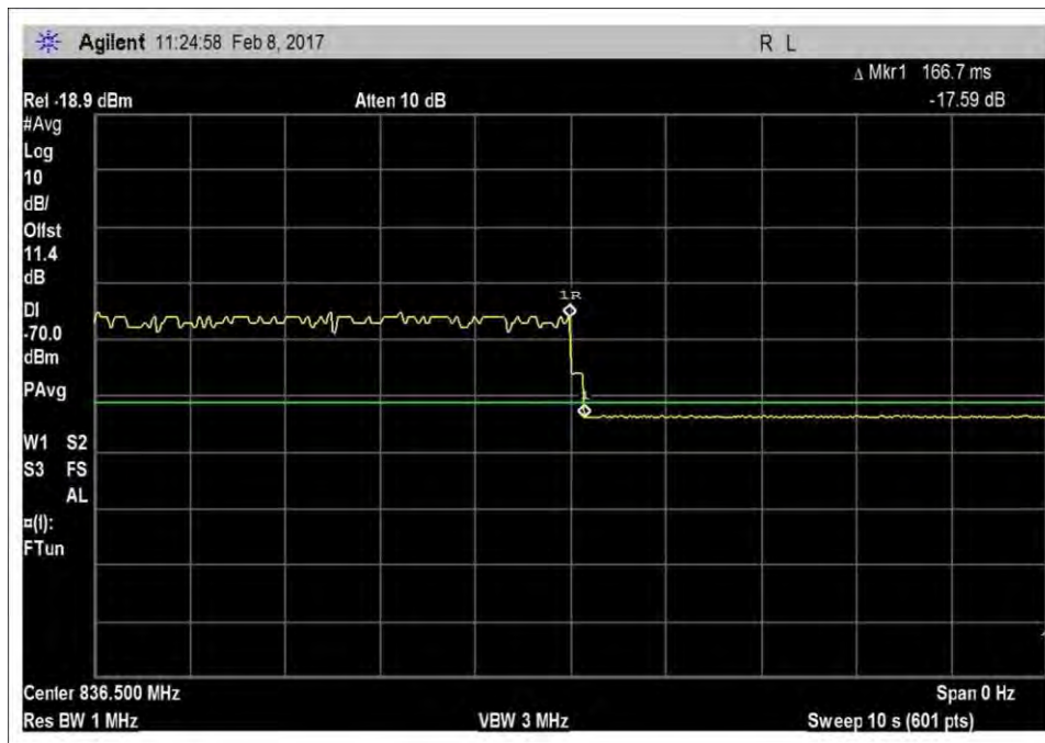
7.7.2_VarNoise_UL_824-849MHz
