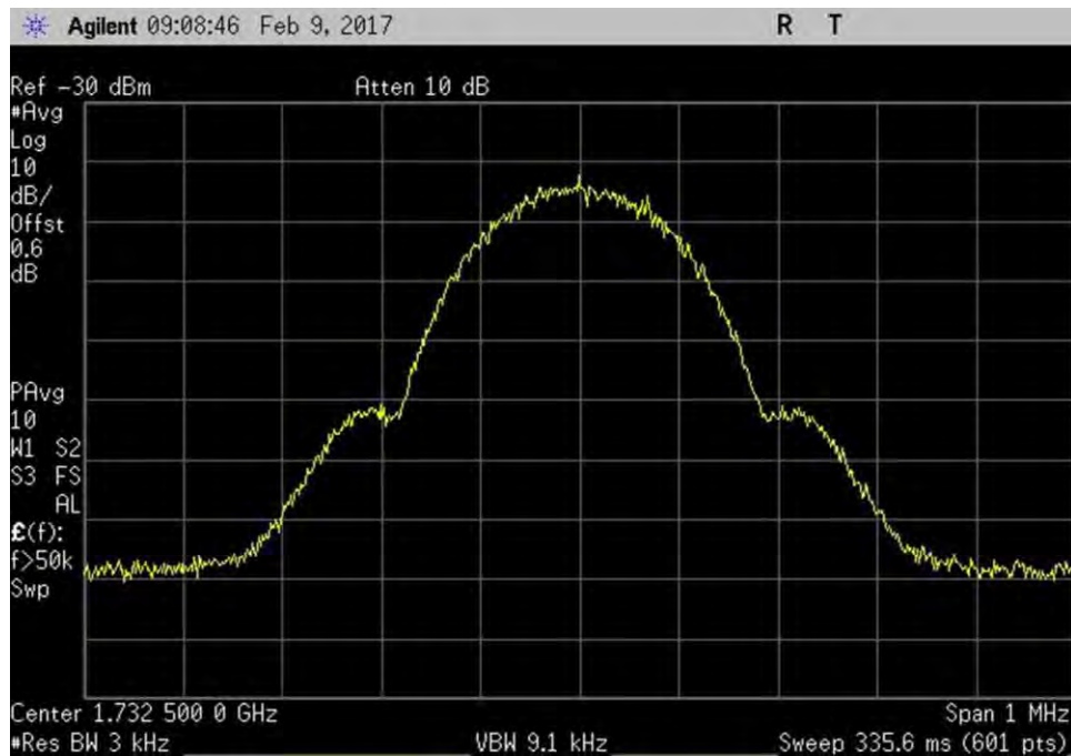
7.10_OBW_UL_1710-1755MHz_GSM_In
