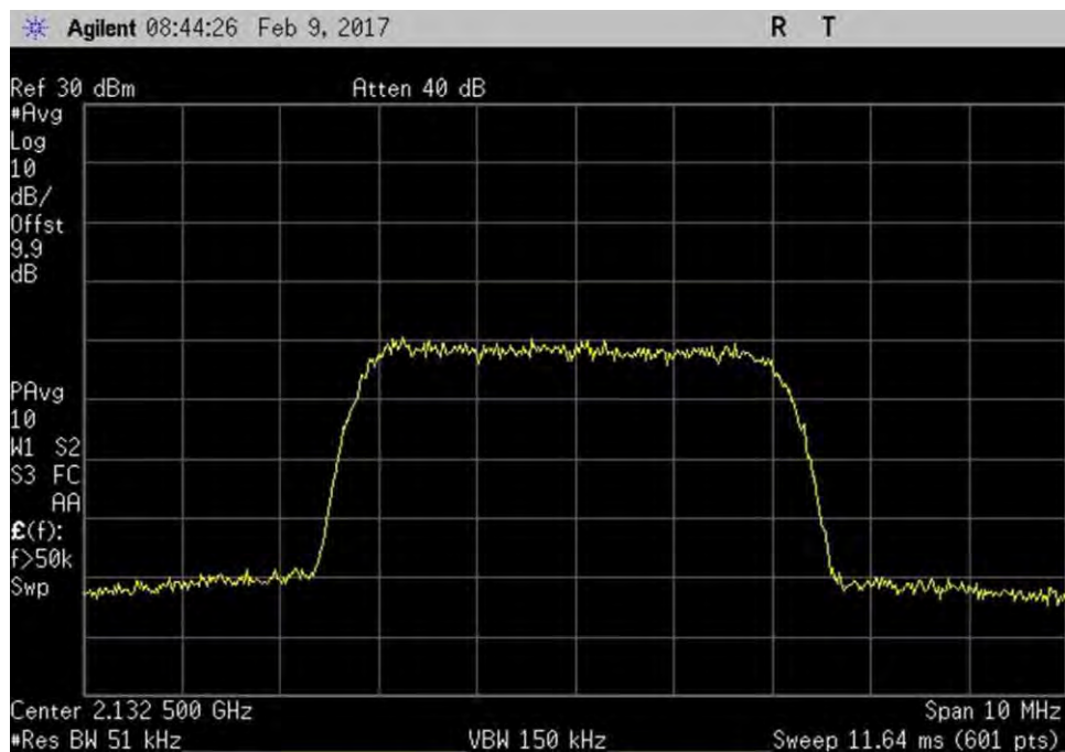
7.10_OBW_DL_2110-2155MHz_WCDMA_Out
