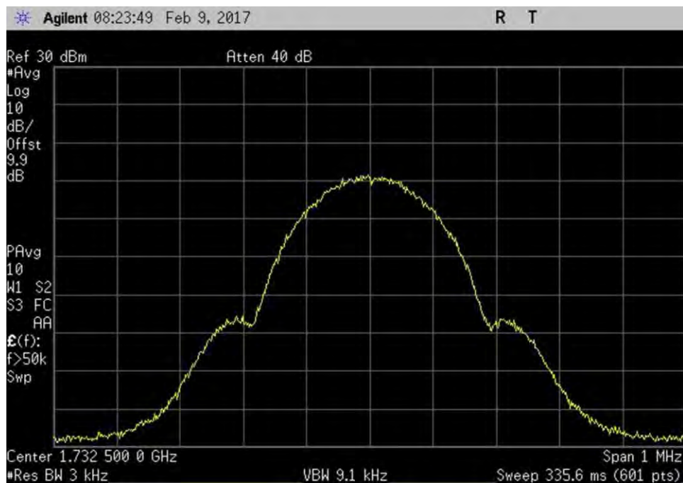
7.10_OBW_UL_1710-1755MHz_GSM_Out
