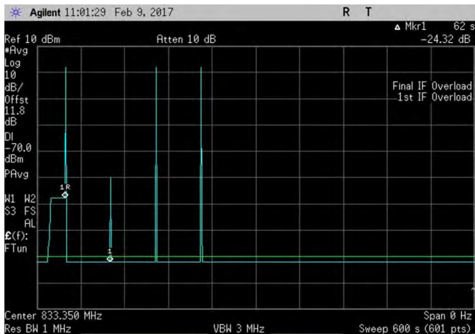
7.11.2_osc_UL_824-849MHz600sec
