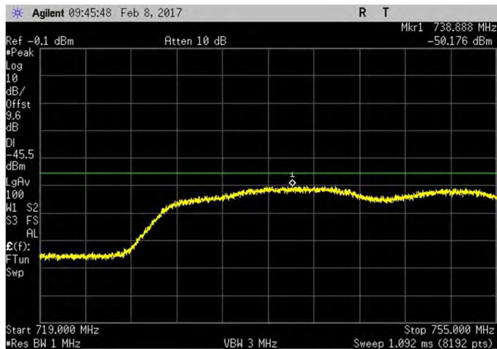
7.7.1_Noise_DL_728-746MHz
