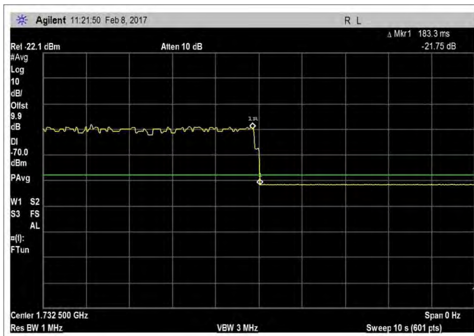
7.7.2_VarNoise_UL_1710-1755MHz
