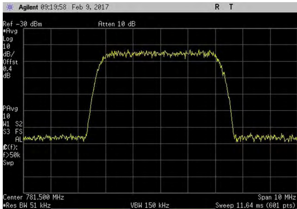
7.10_OBW_UL_776-787MHz_WCDMA_In
