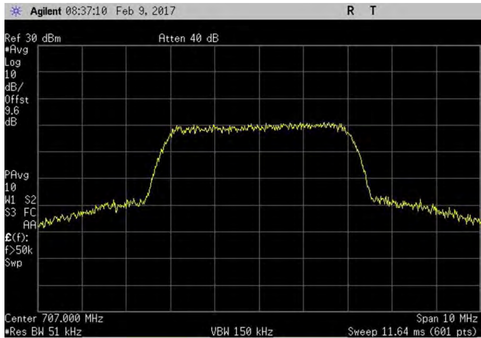
7.10_OBW_UL_698-716MHz_WCDMA_Out
