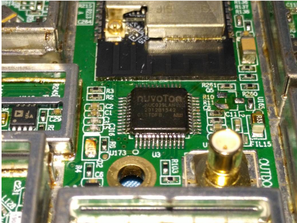
Wi-Fi Module
